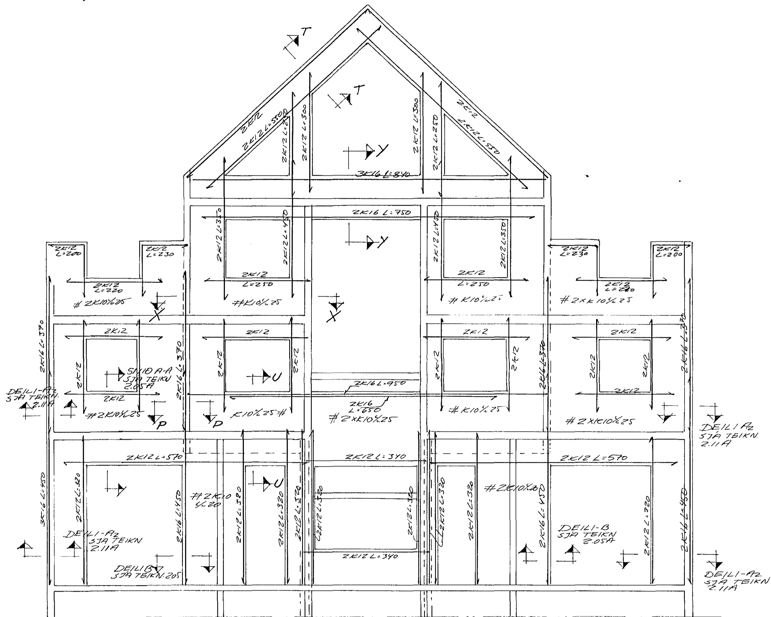
VEGGUR-V3 1:50
