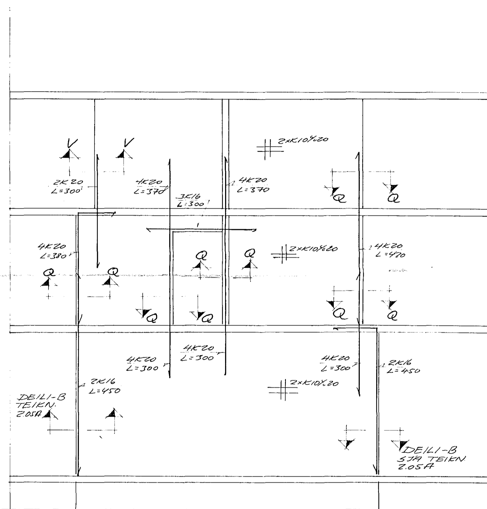
VEGGUR-V4 1:50
