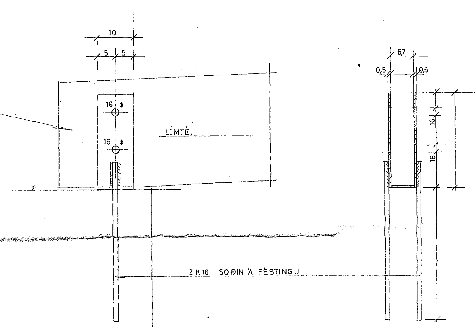
FESTING SPERRU VIÐ VEGG A ÞVOTTARSTÖÐ MK 1:5
