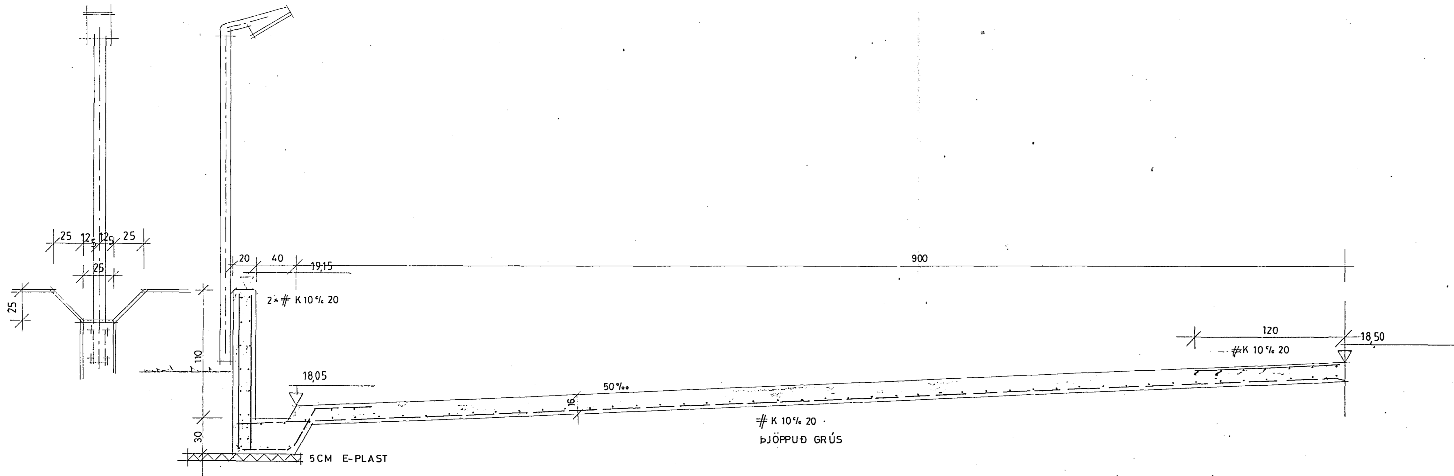
SNIÐ H-H 1:20
