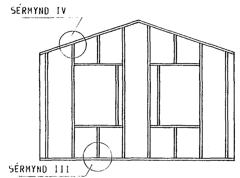
NORÐUR HLIÐ
