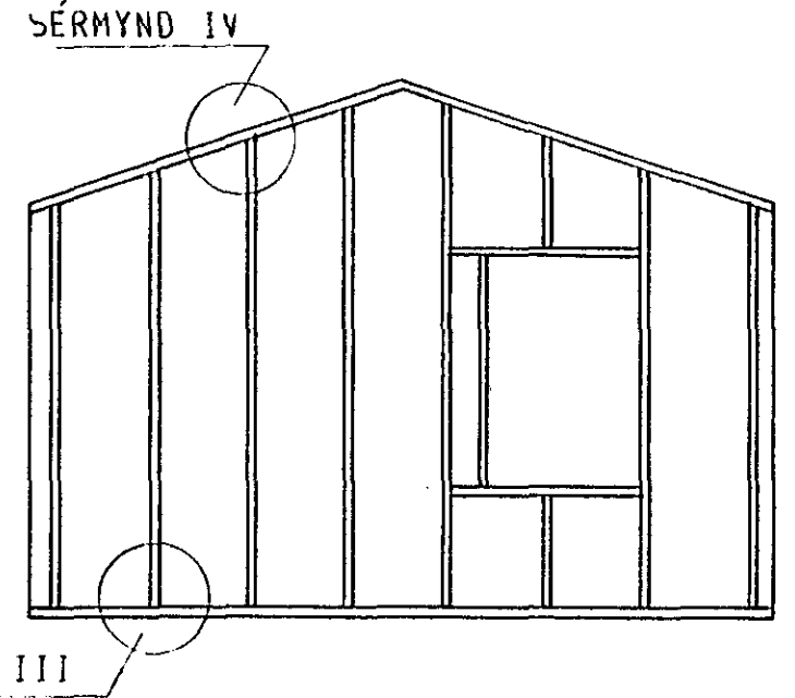
SUÐUR HLIÐ
