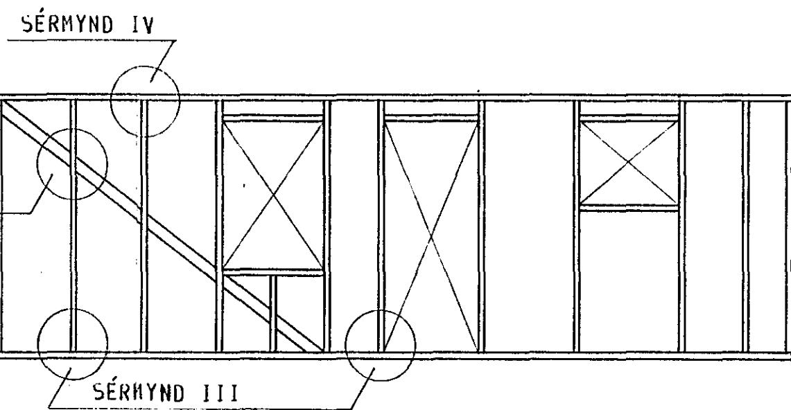
VESTUR HLIÐ
