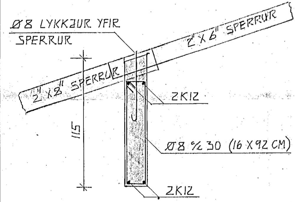
SNID I-I
