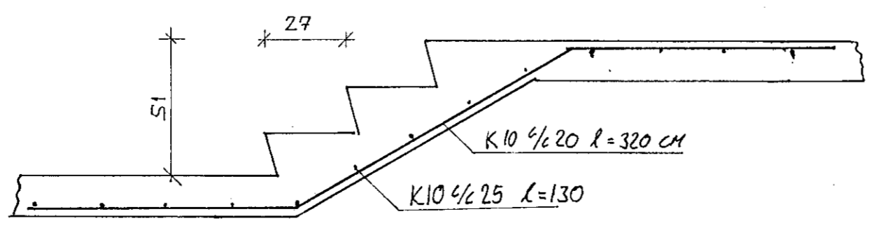
SNEIDING A-A M 1:20
