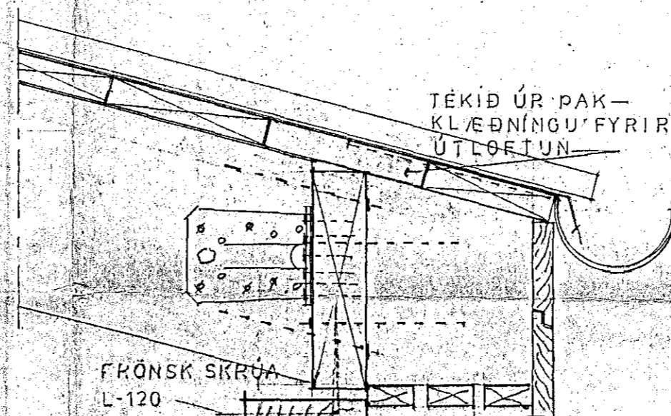
SNEIDING A-A
