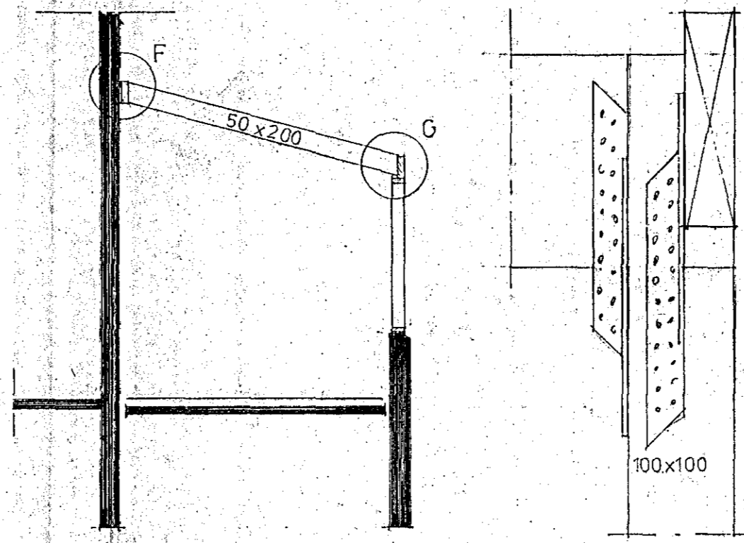
SNEIDING A-A
