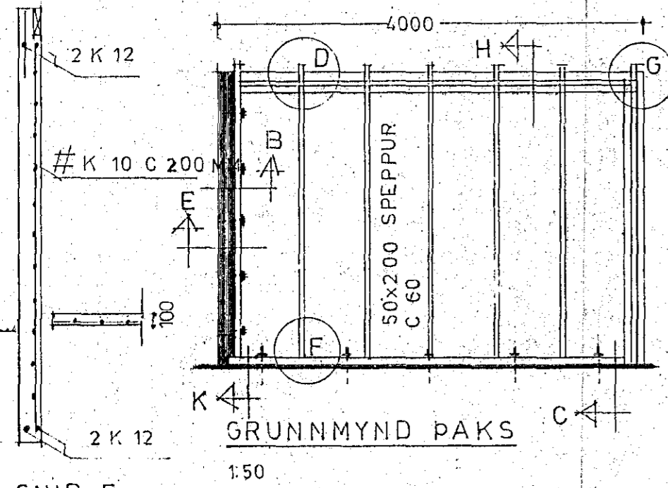
SNID E 1:50
