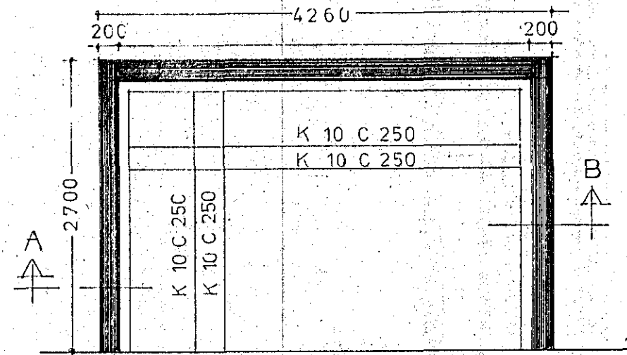
GRUNNMYND PLÖTU 1:50
