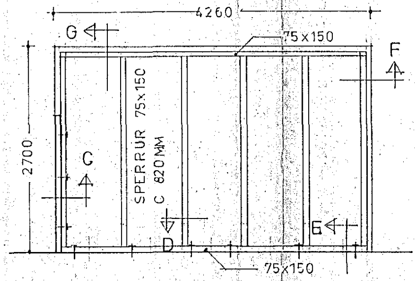
GRUNNMYND ÞAK 1:50
