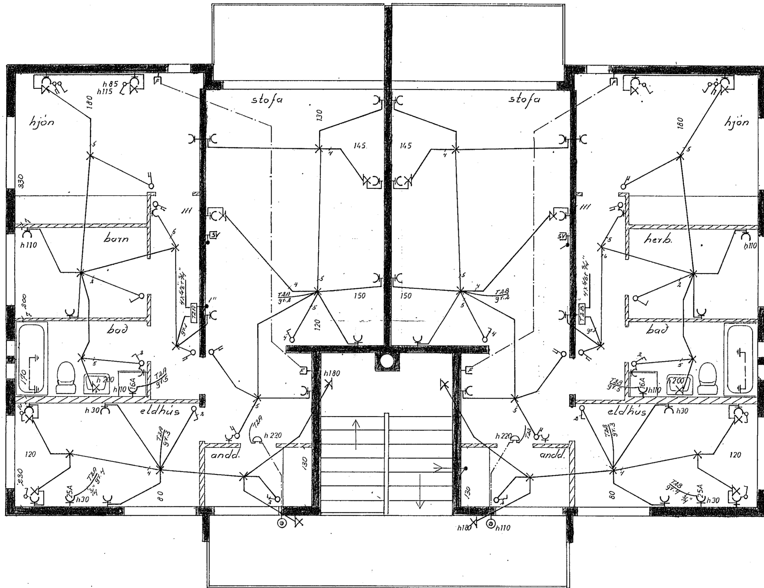
2. hæð
