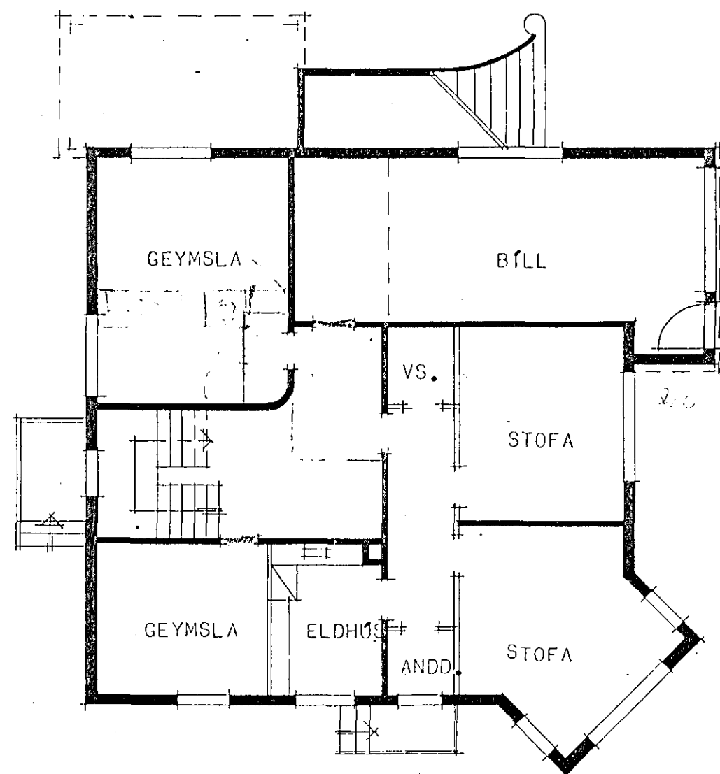
GRUNNMYND KJALLARA
