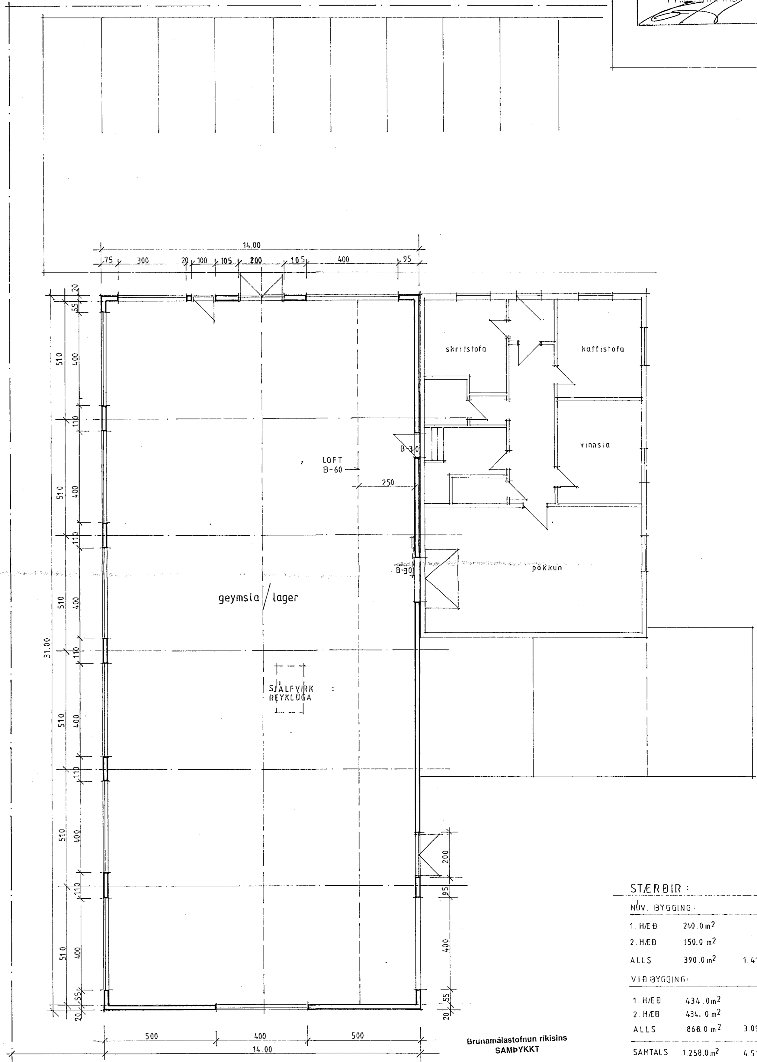
GRUNNMYND EFRI HÆÐ
