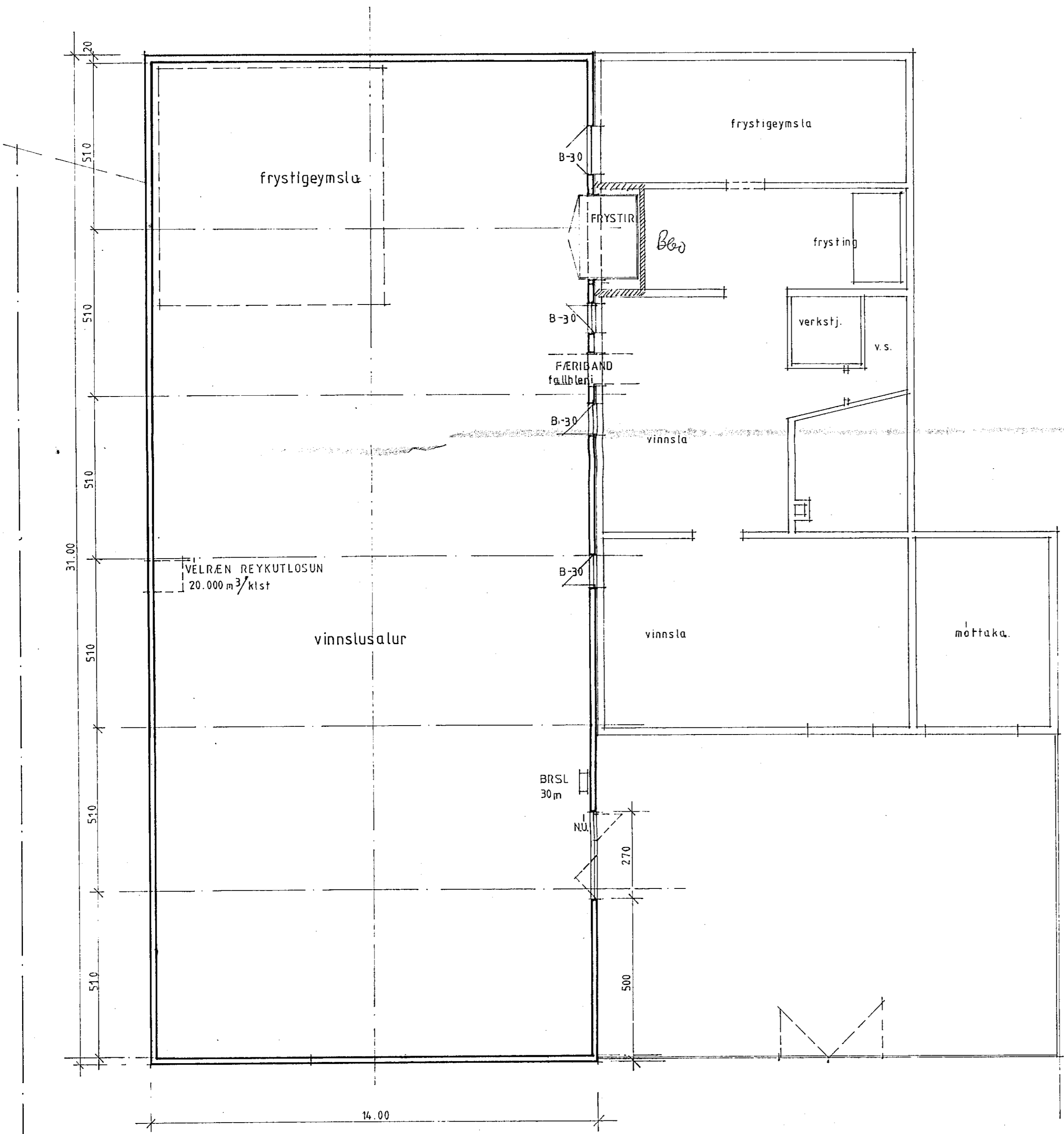
GRUNNMYND NEDRI HÆÐ
