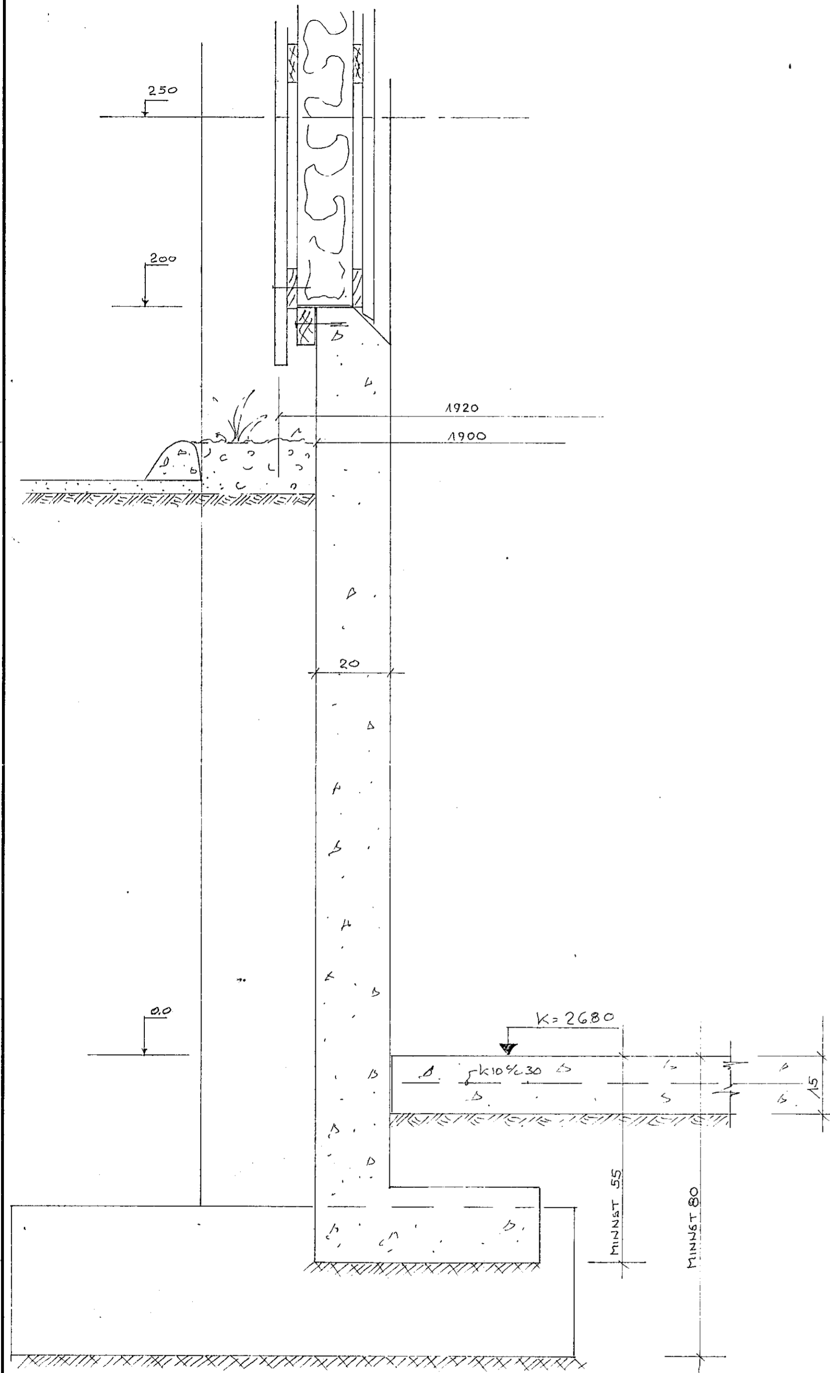
SNID Í VEGG 1:10
