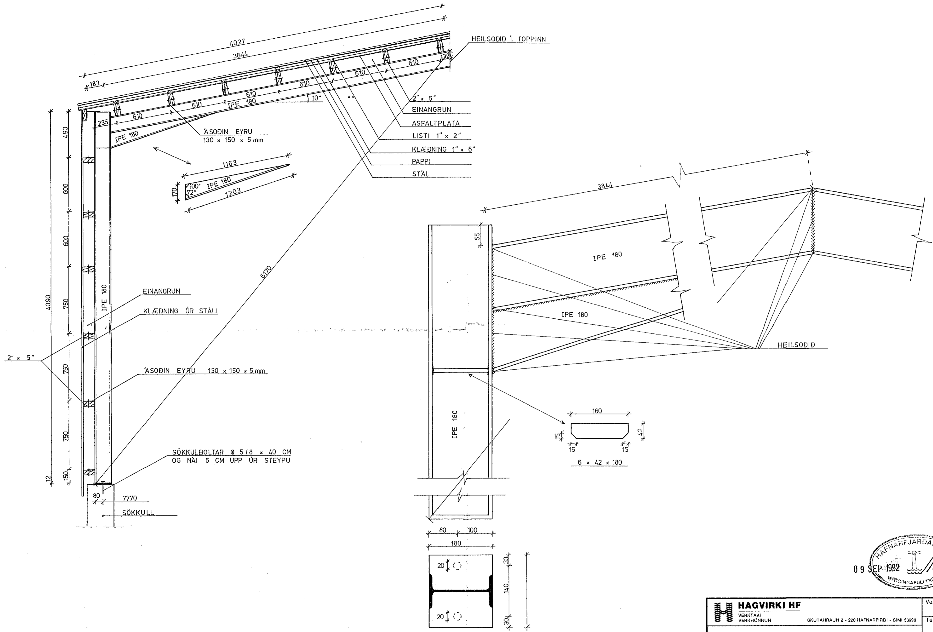
FÓTPLATA 200 x 180 x 12 MKV. 1 : 5
