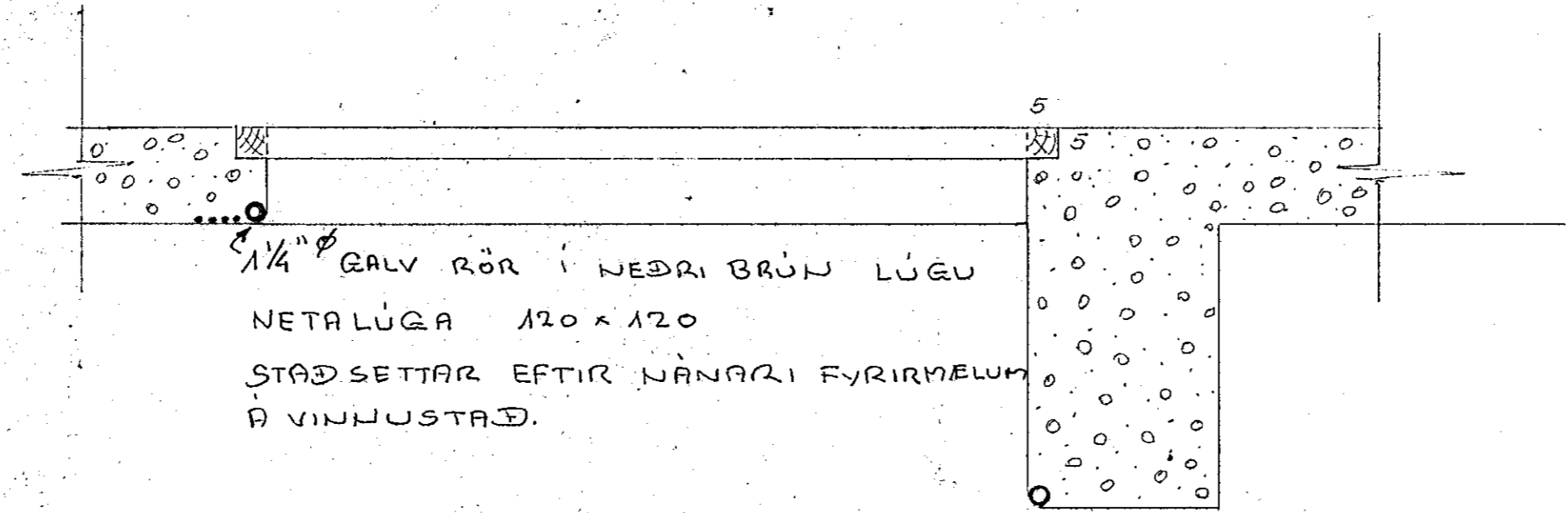
FRÁGANGUR NETALÚGU 1:10
