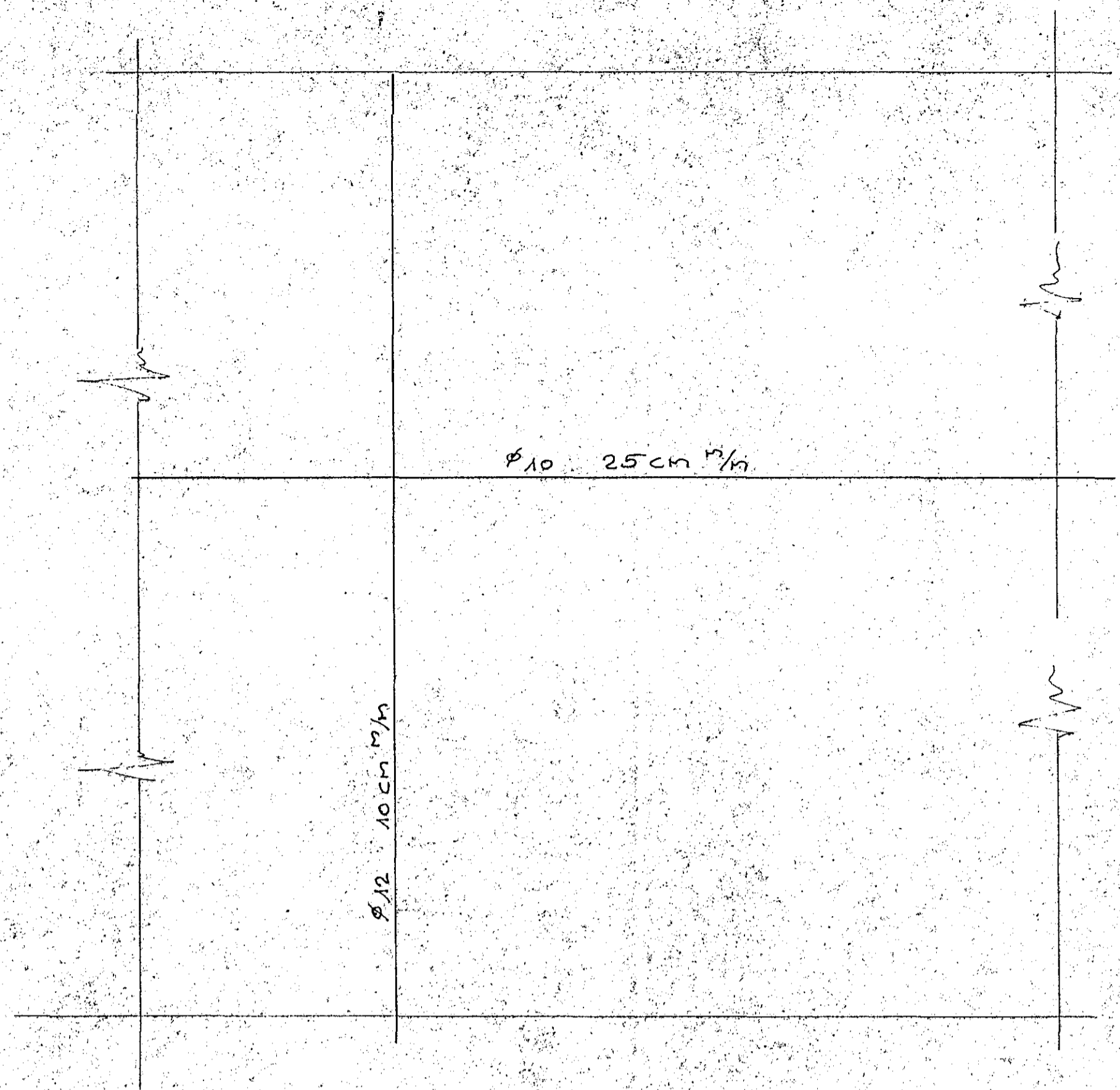
JÄRNALÖGN I VEGGI, SEM Fyllt er uppáð 1:20
