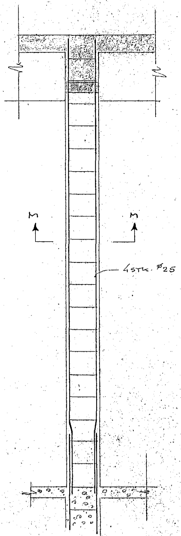
SÚLA M=1:20
