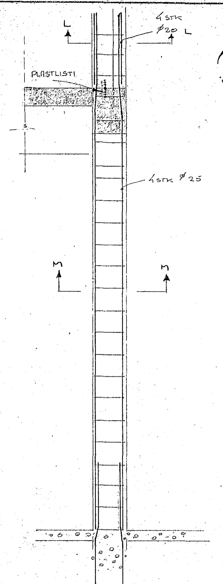
VEGG SÚLA M=1:20
