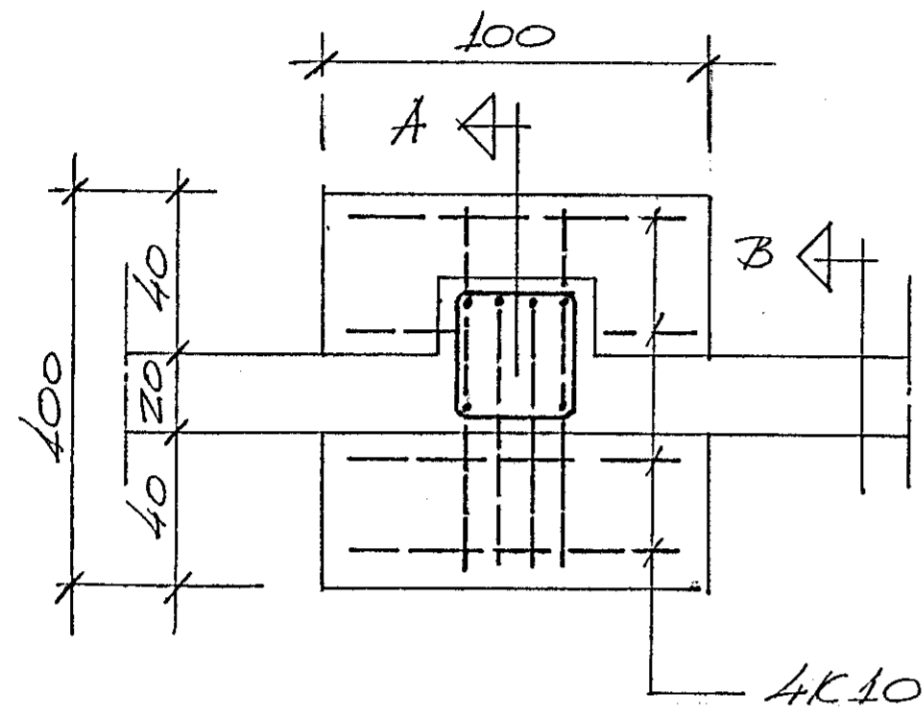
GRUNNMYND SÚLUUNDIRSTÖÐU
