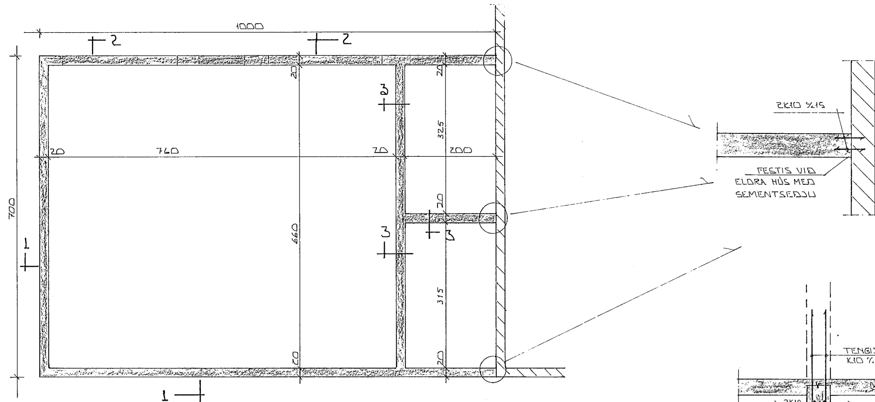
GRUNNMYND UNDIRSTÖÐUR ~1:50
