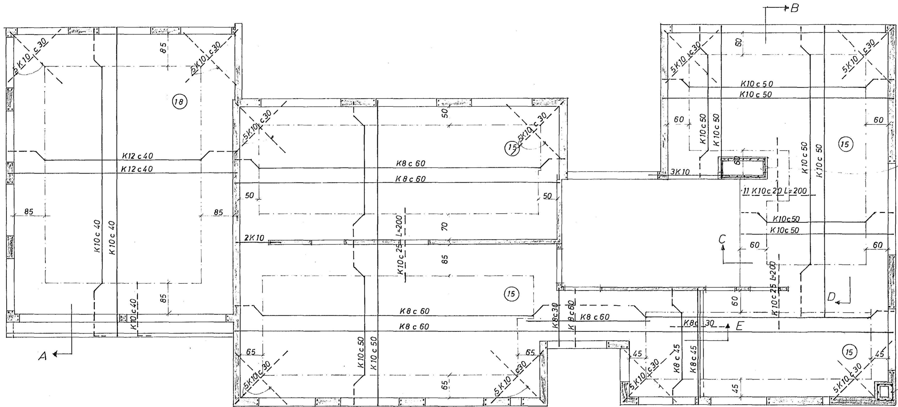
GRUNNMYND 1:50
