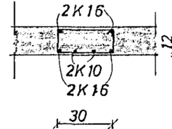
SNID D 1:20
