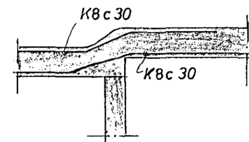
SNID E 1:20
