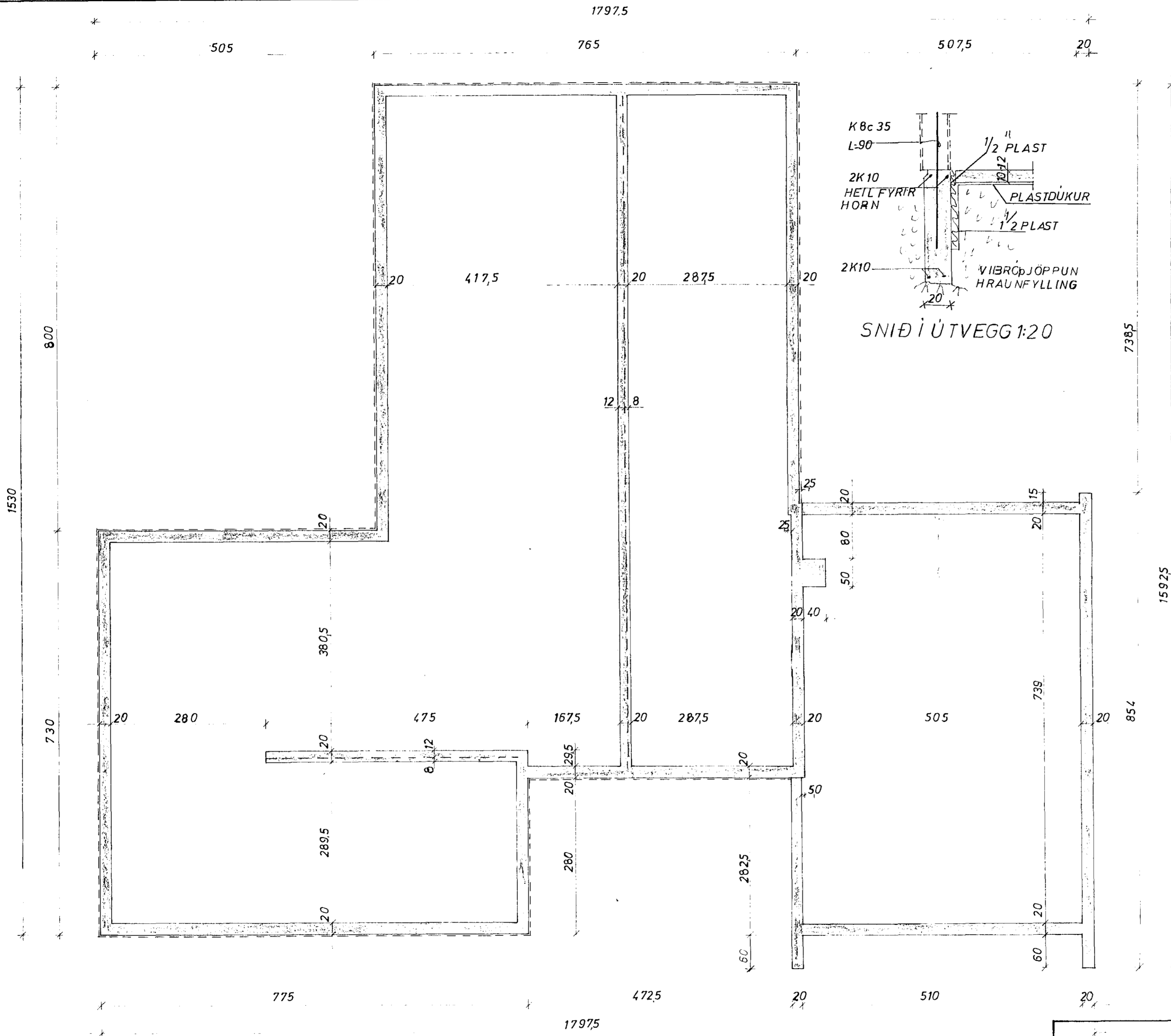
GRUNNMYND 1:50
