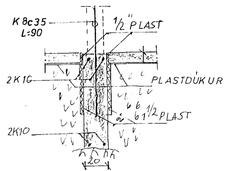
SNIDÍ INNVEGG 1:20
