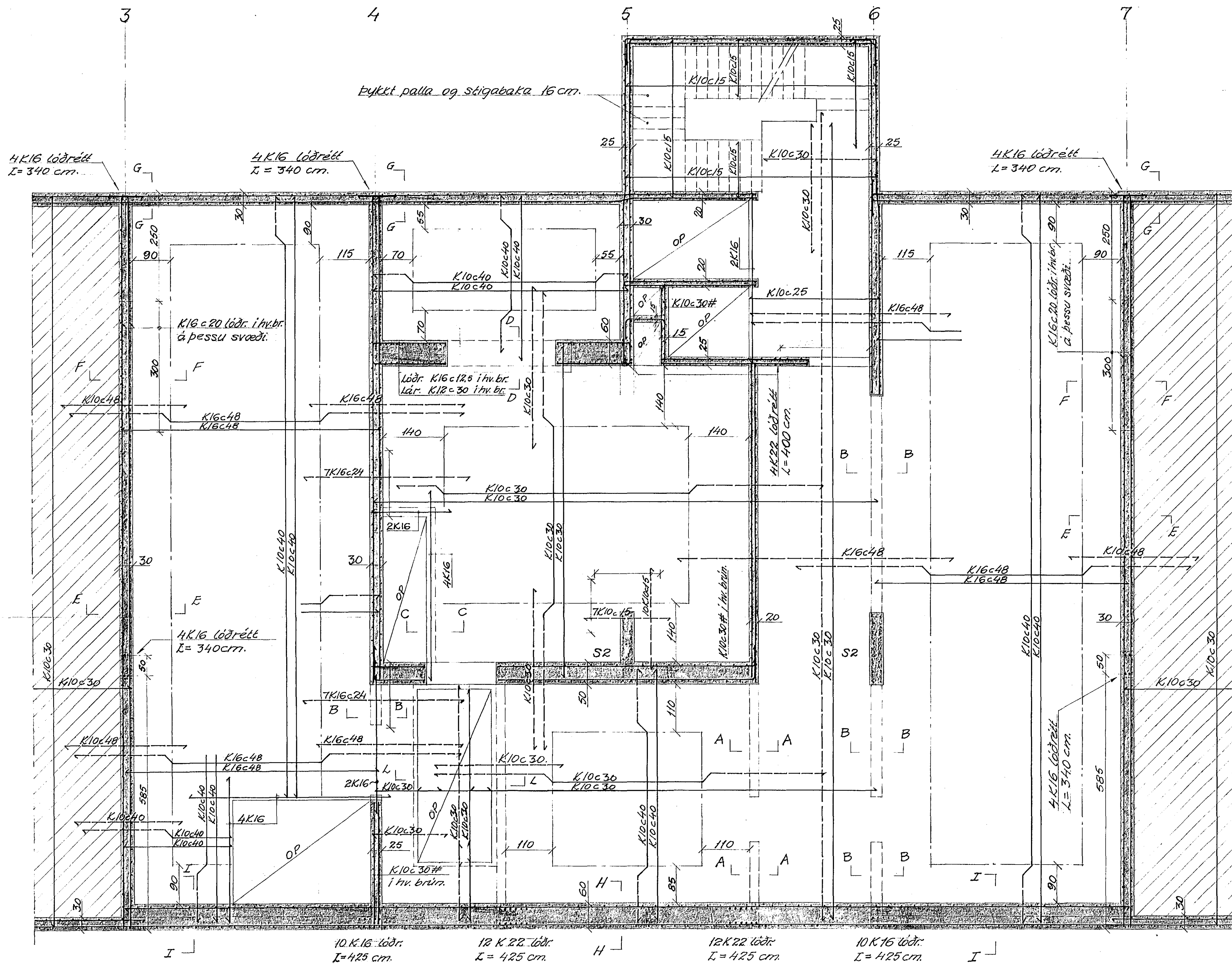
Grunnmynd 1:50
