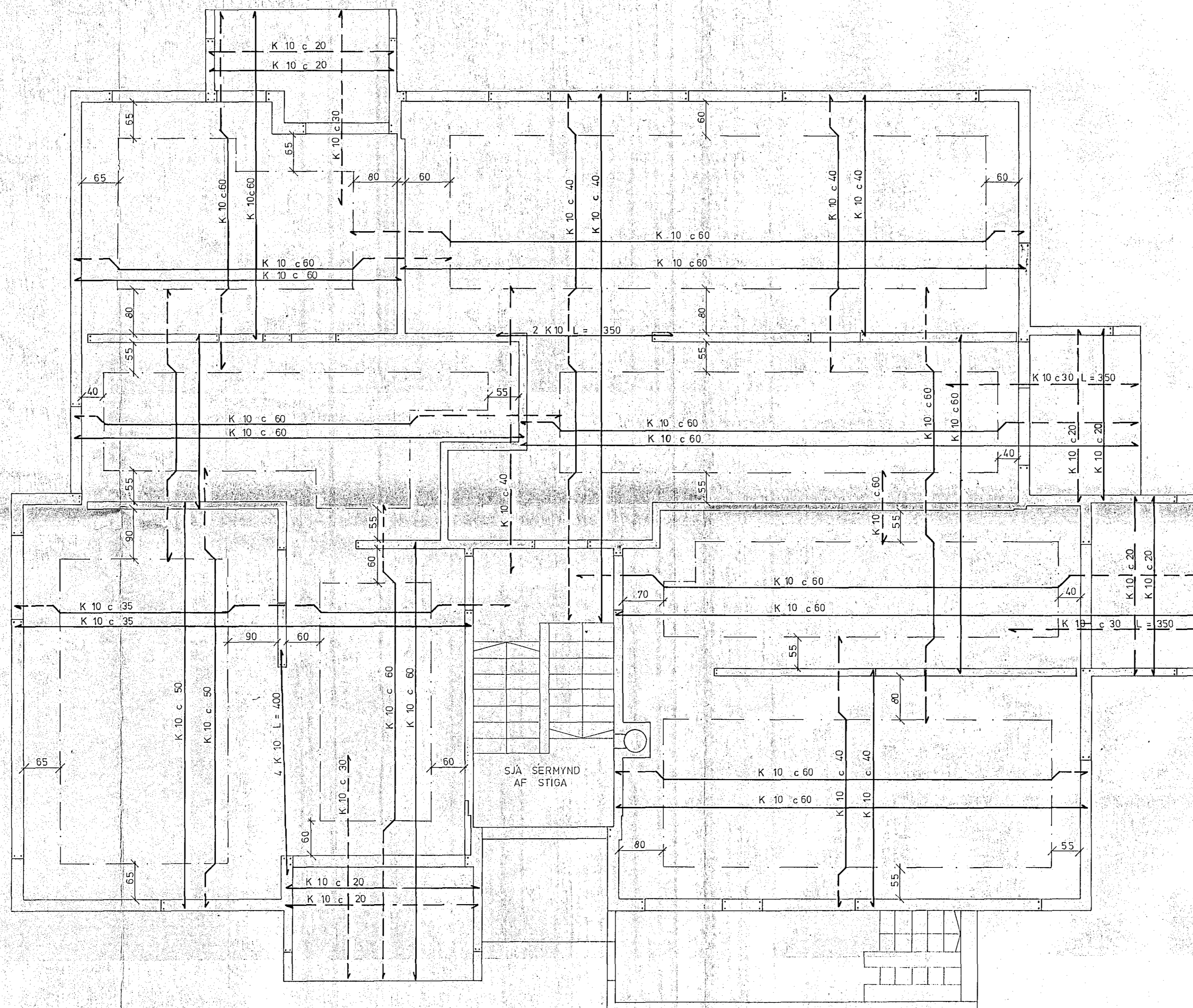
GRUNNMYND 1 HÆÐAR 1:50
