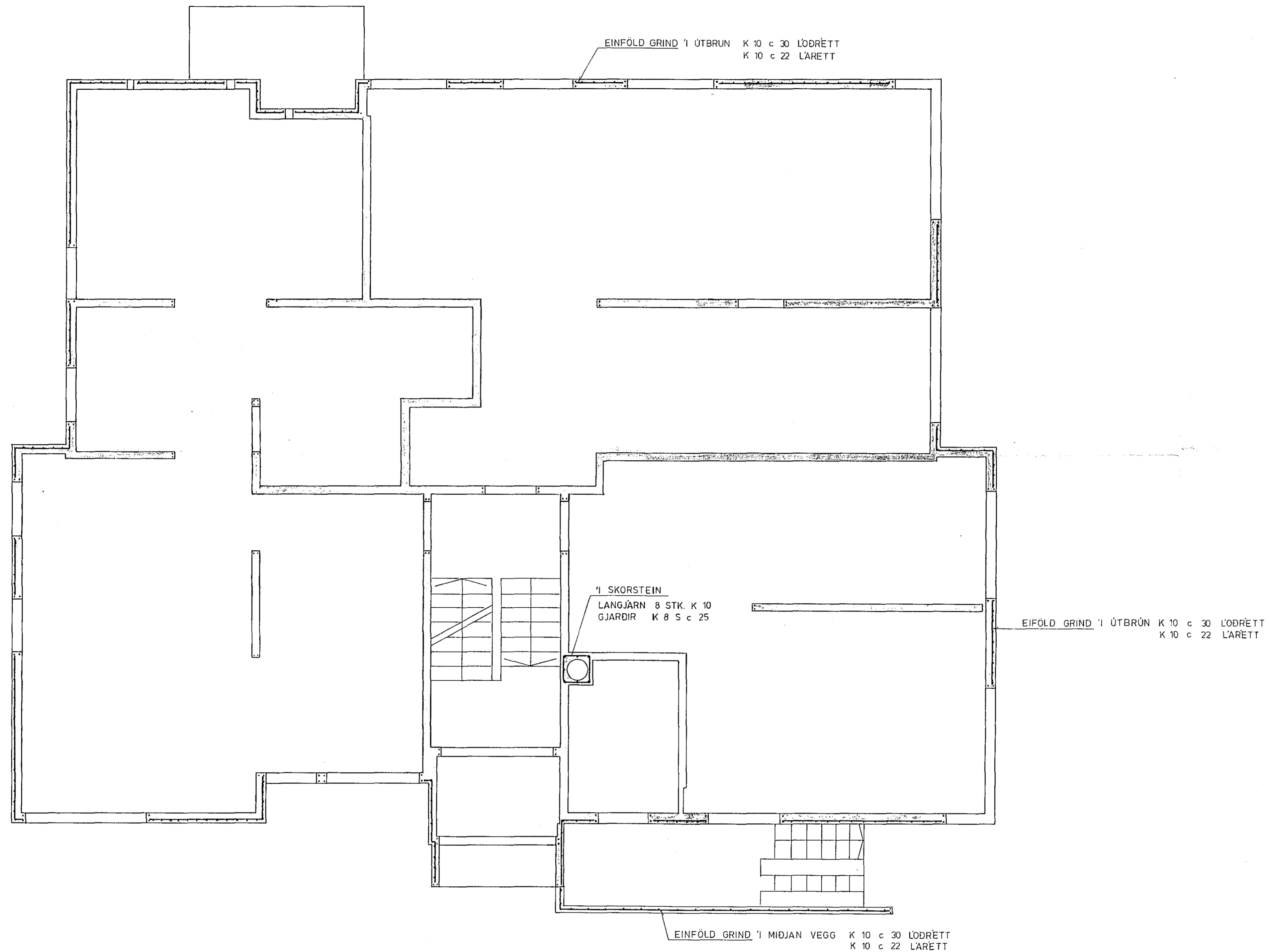
GRUNNMYND KJALLARA 1 : 50
