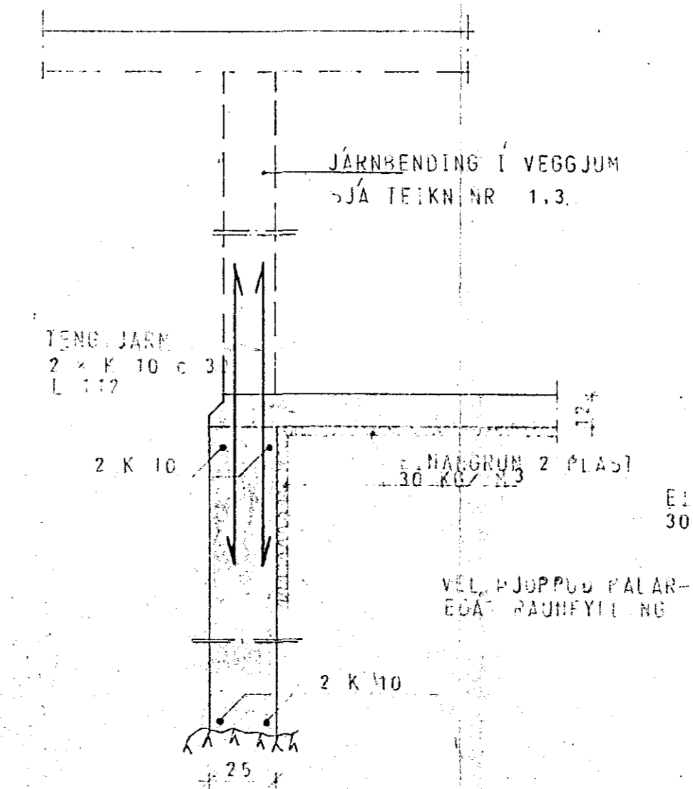
SNID D 1:20
