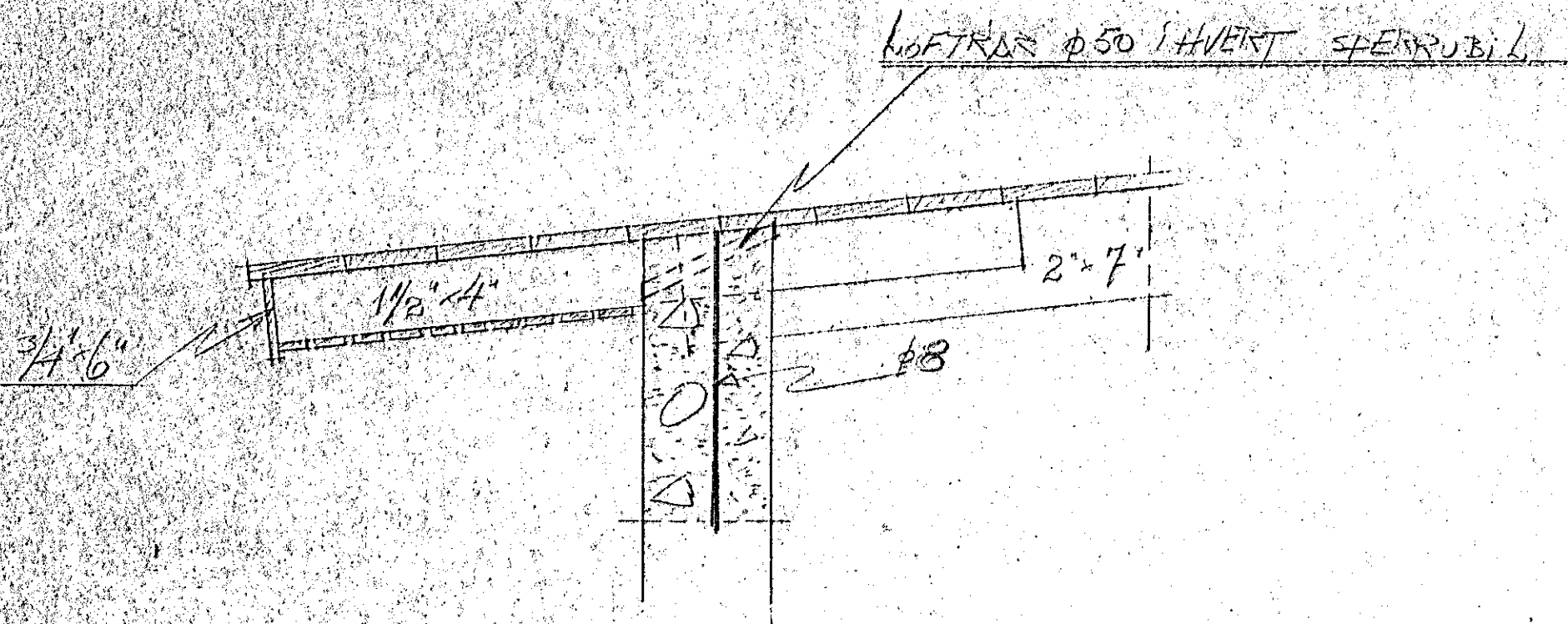
SNITT - E KVAFI 1:10
