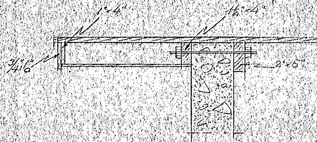
SNITT - D KVAFI 1:10
