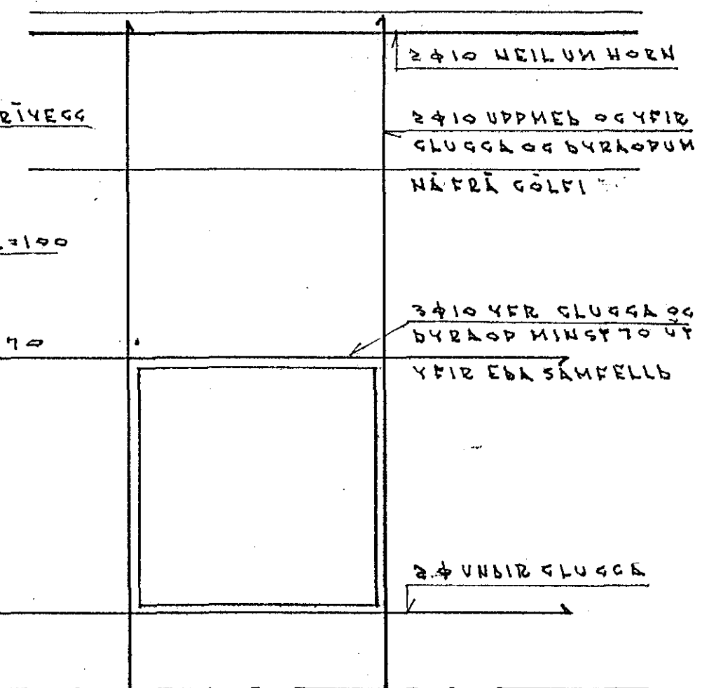
YFIR KEING MÜRÖP M 1:20
