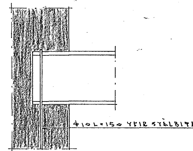
SNIB VIBVEGG M 1:5
