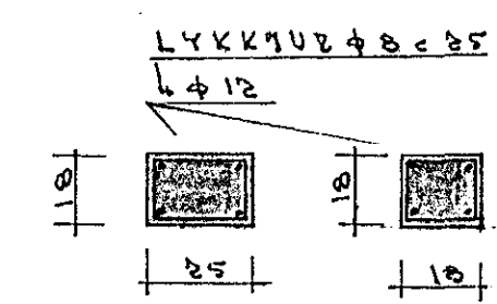
SÜLA 51 OG 52 1:20
