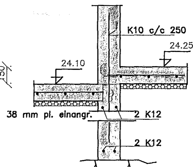
SNID B-B 1:20
