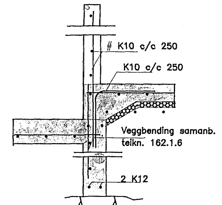
SNID D-D 1:20
