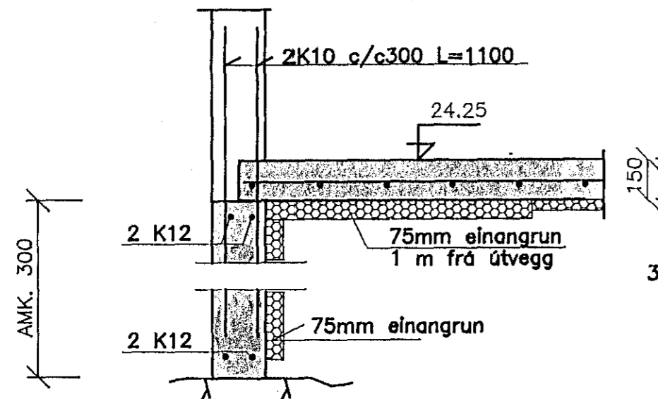
SNID A-A 1:20
