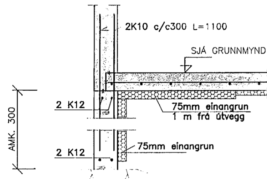
SNID A-A 1:20
