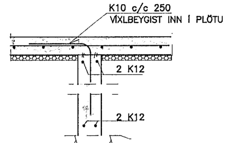
SNID G-G 1:20
