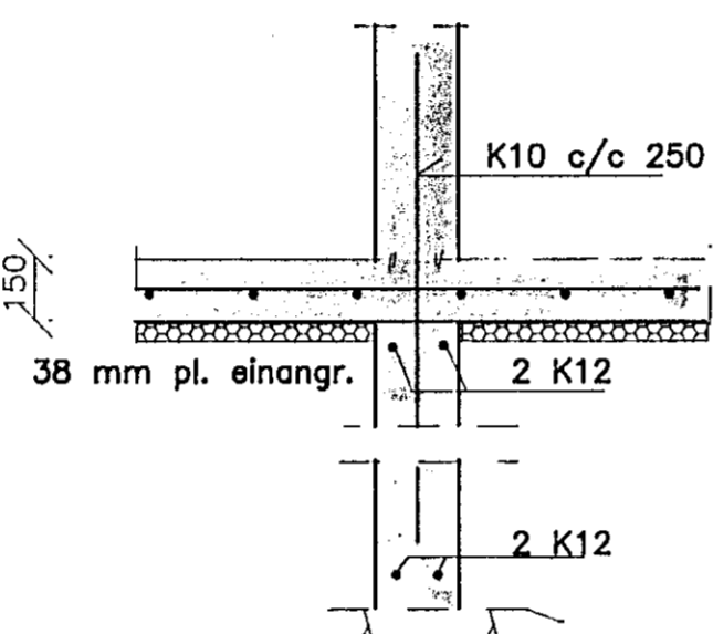
SNID B-B 1:20
