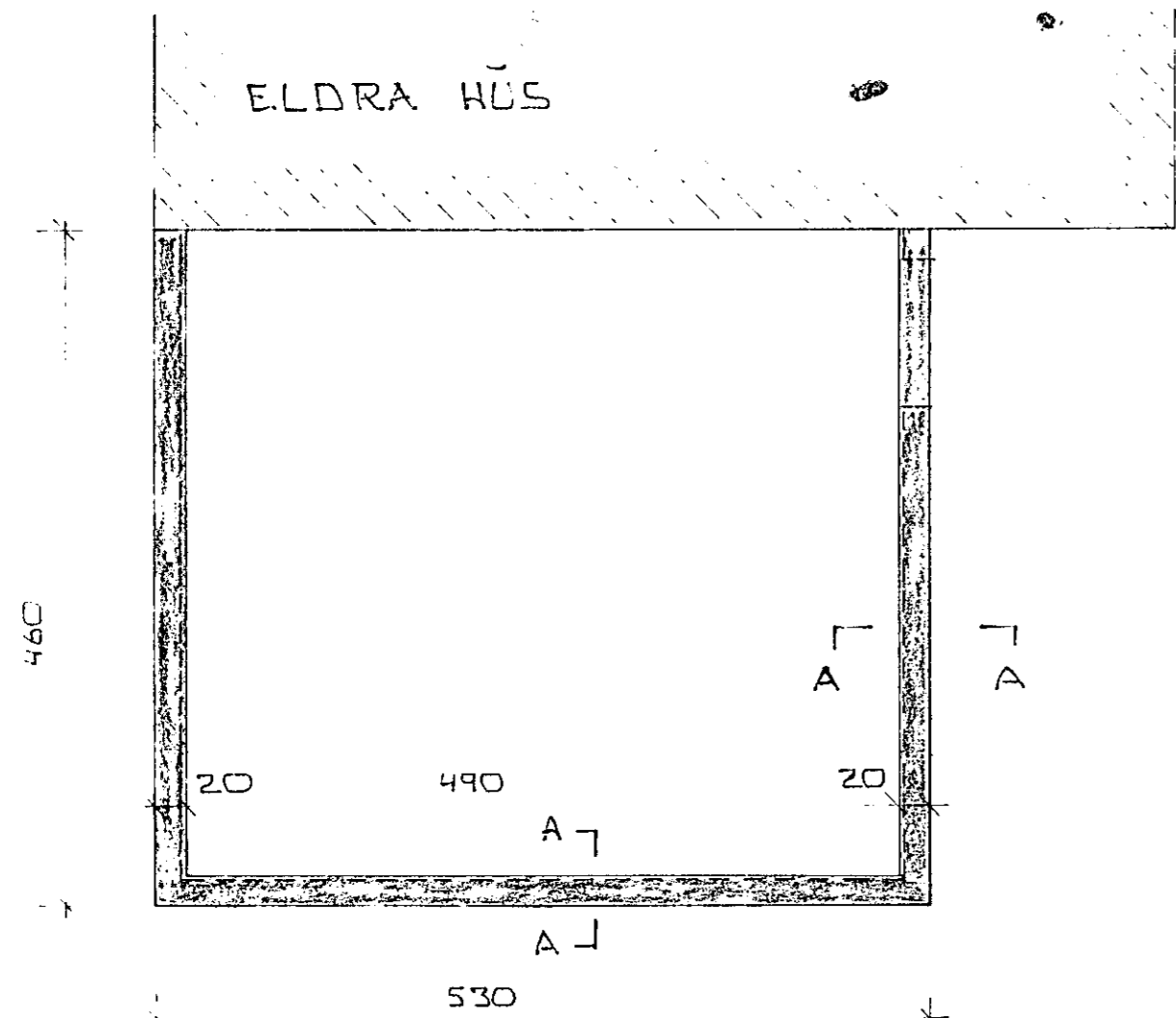
GRUNNMYND UNDIRSTÖÐUR 1:50
