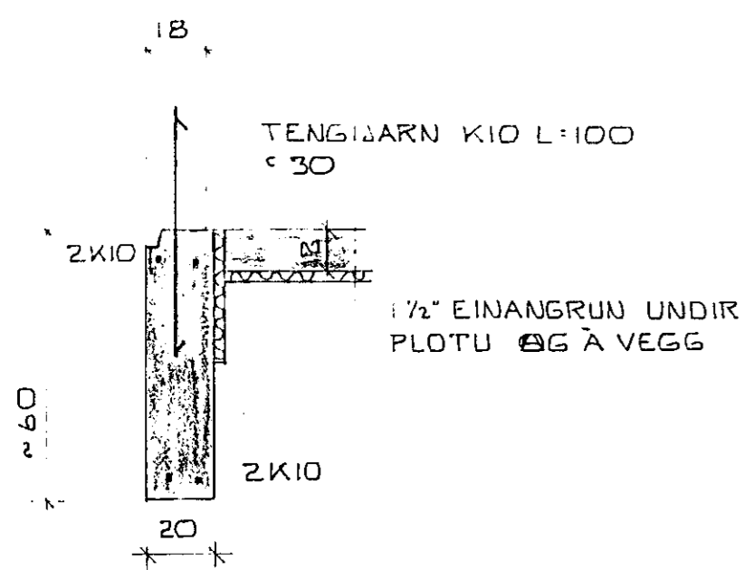
SNID A-A 1:20
