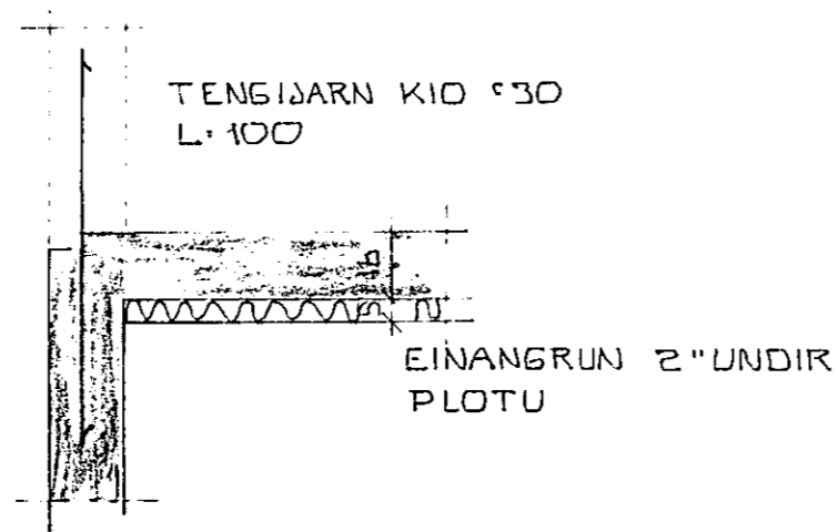
SNID B-B 1:20
