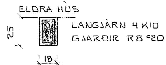
SNID B-B 1:20
