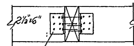
⑦ SNÍÐ
