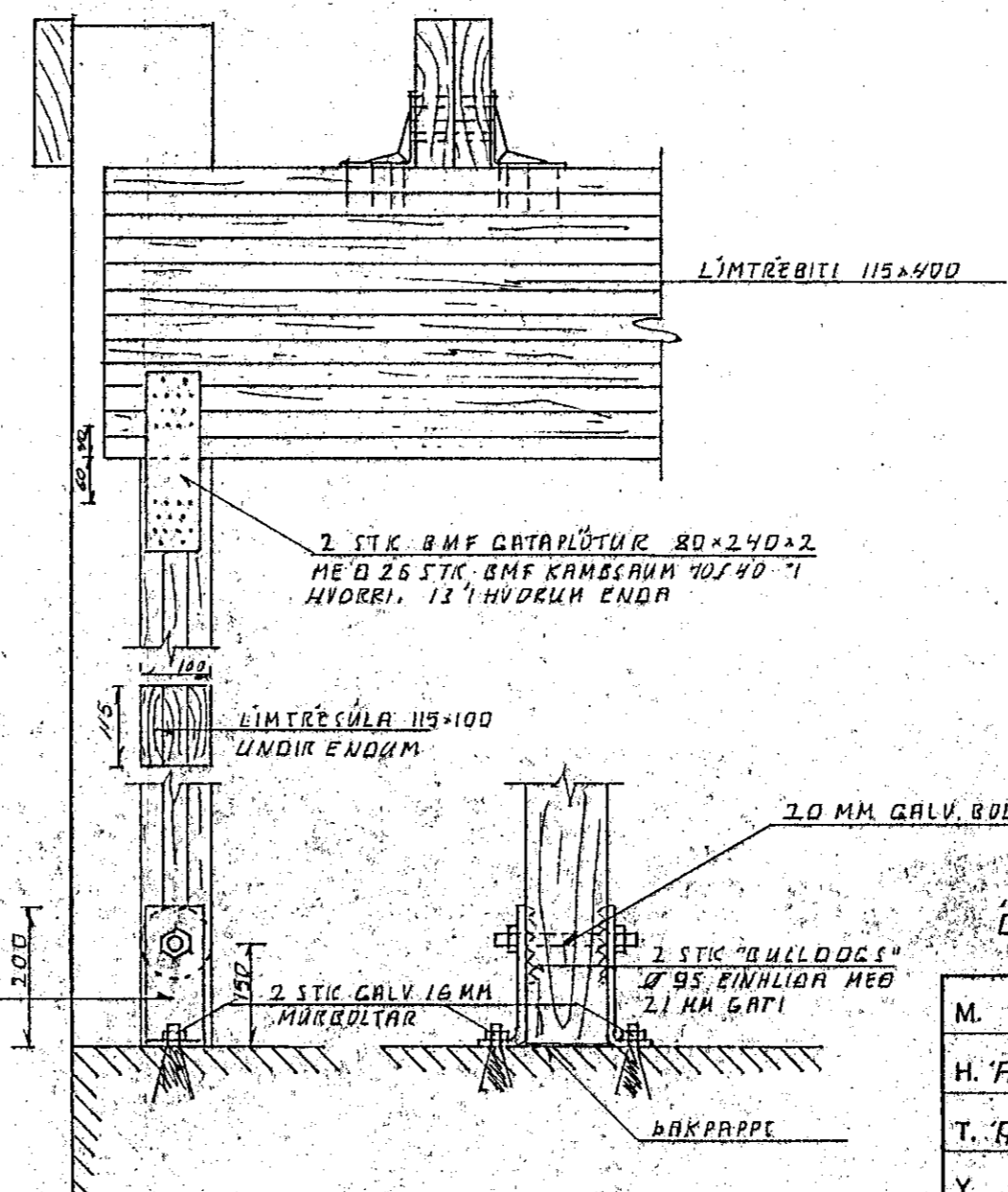
SNÍÐ B-B 1:10
