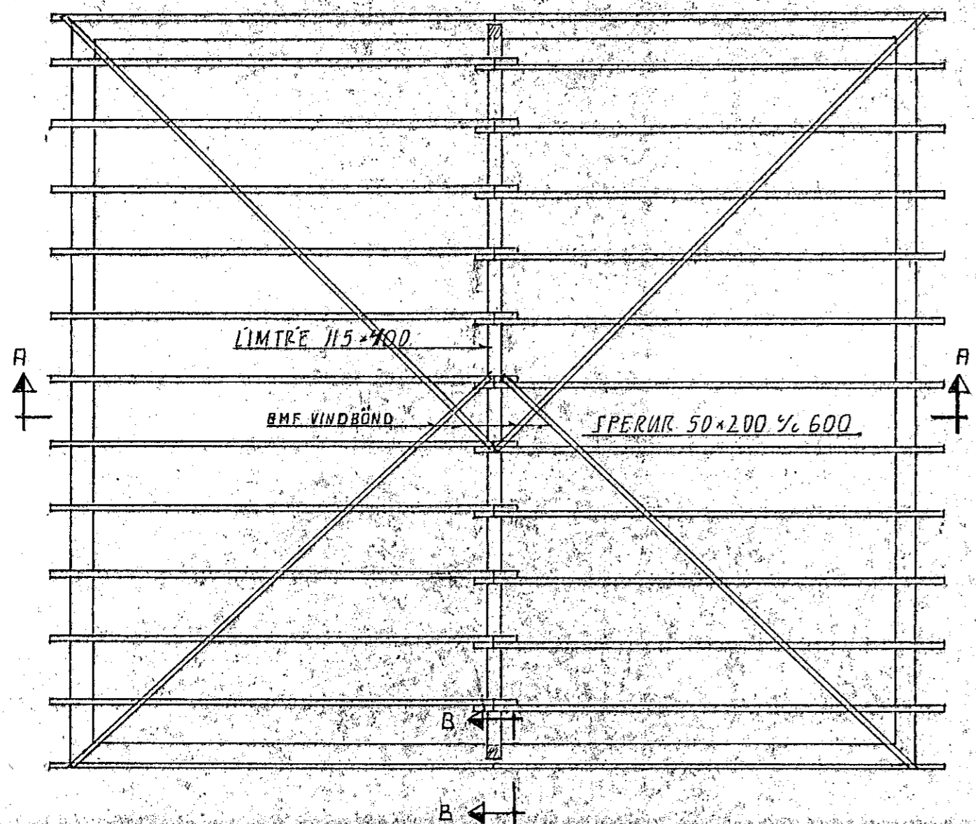
GRUNNMYND 1:50
