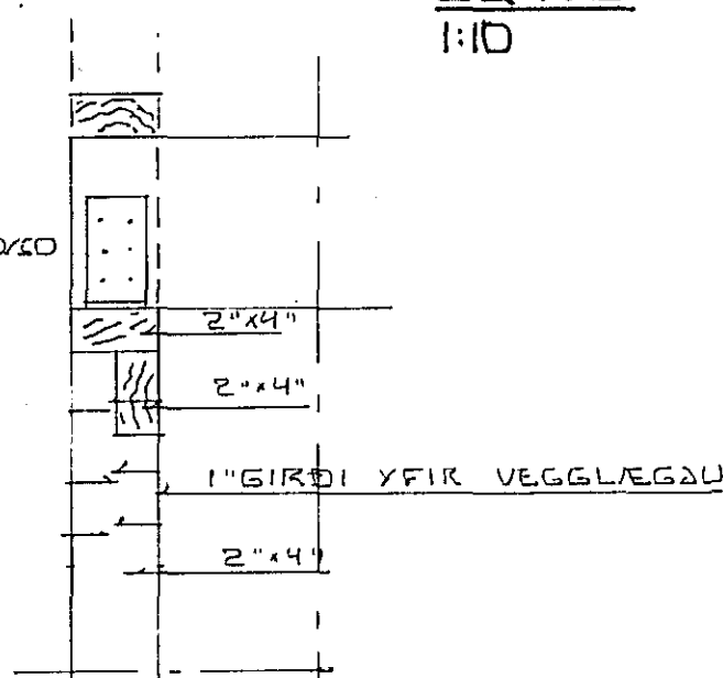
SNID A-A 1:10
