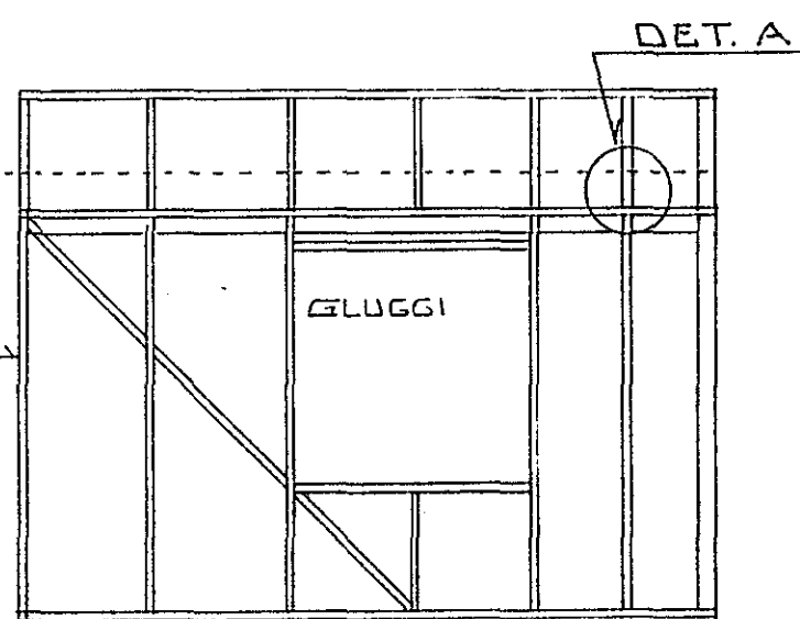
VEGGGRIND 1:50
