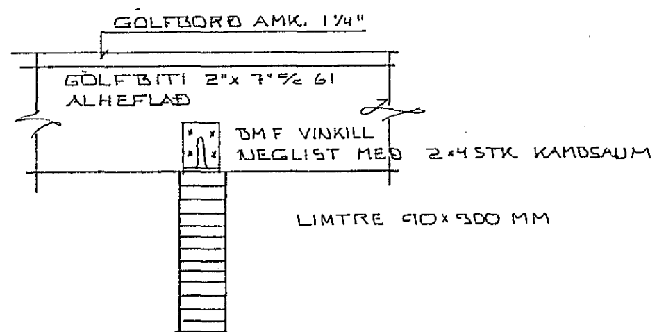
DET. C 1:10
