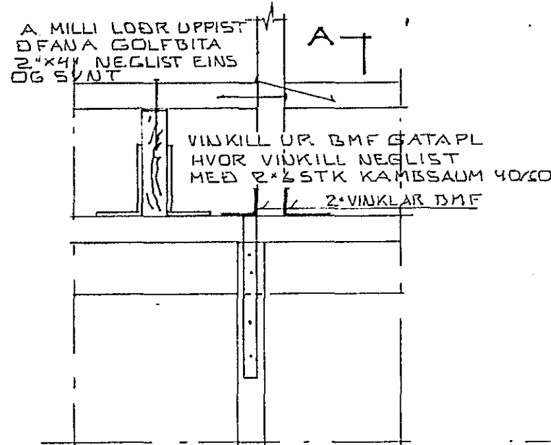
DET. A 1:10
