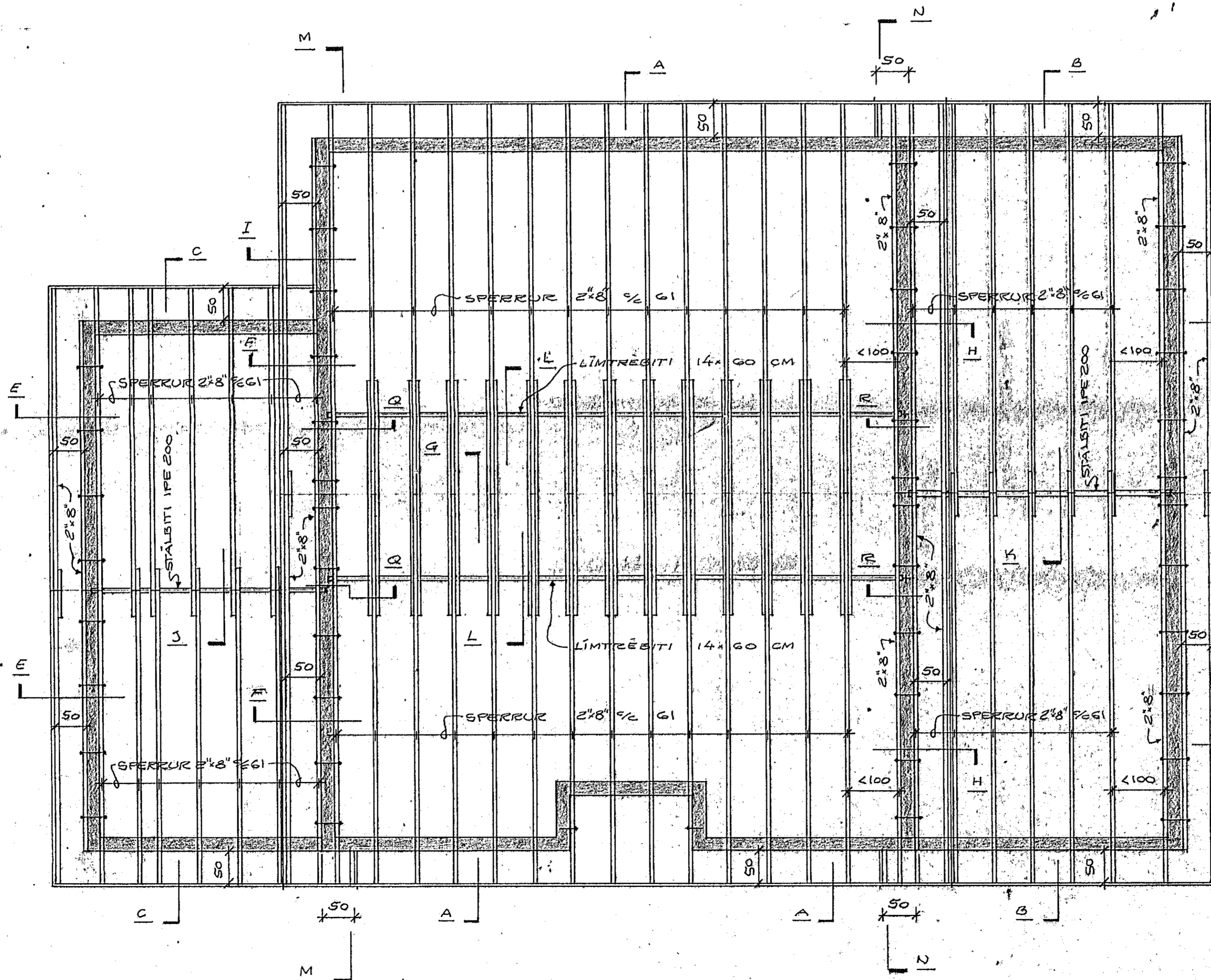
GRUNNMÝND, M=1:50
