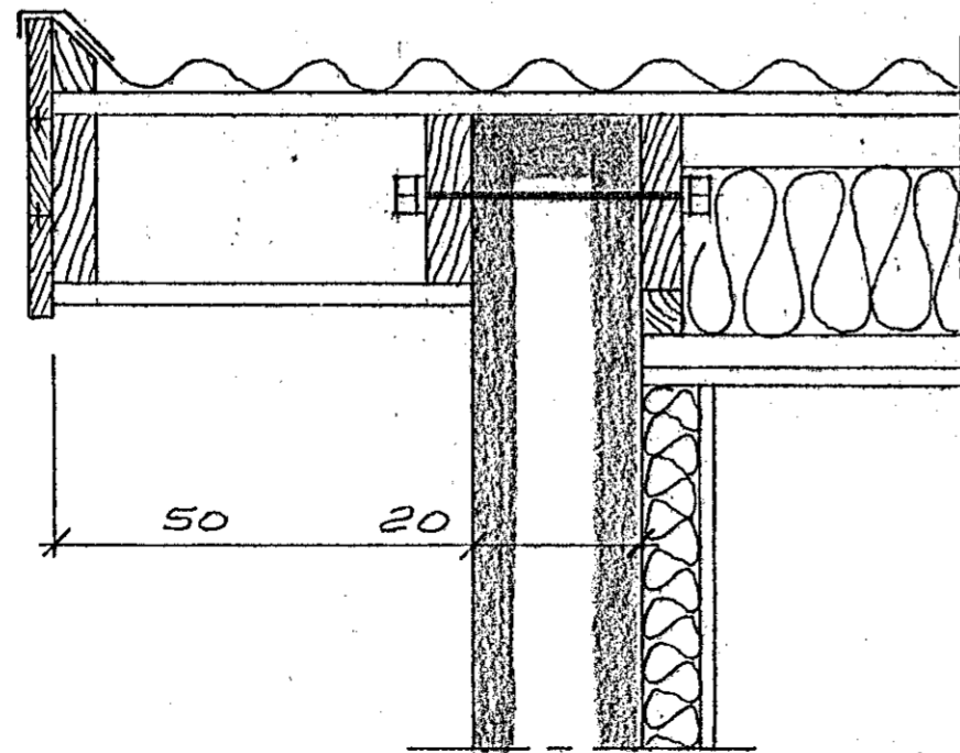
STÄLBITAENDAR Í VEGG, M=1:10
