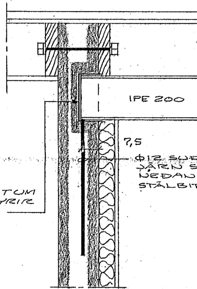
STÄLBITAENDAR Í VEGG, M=1:10
