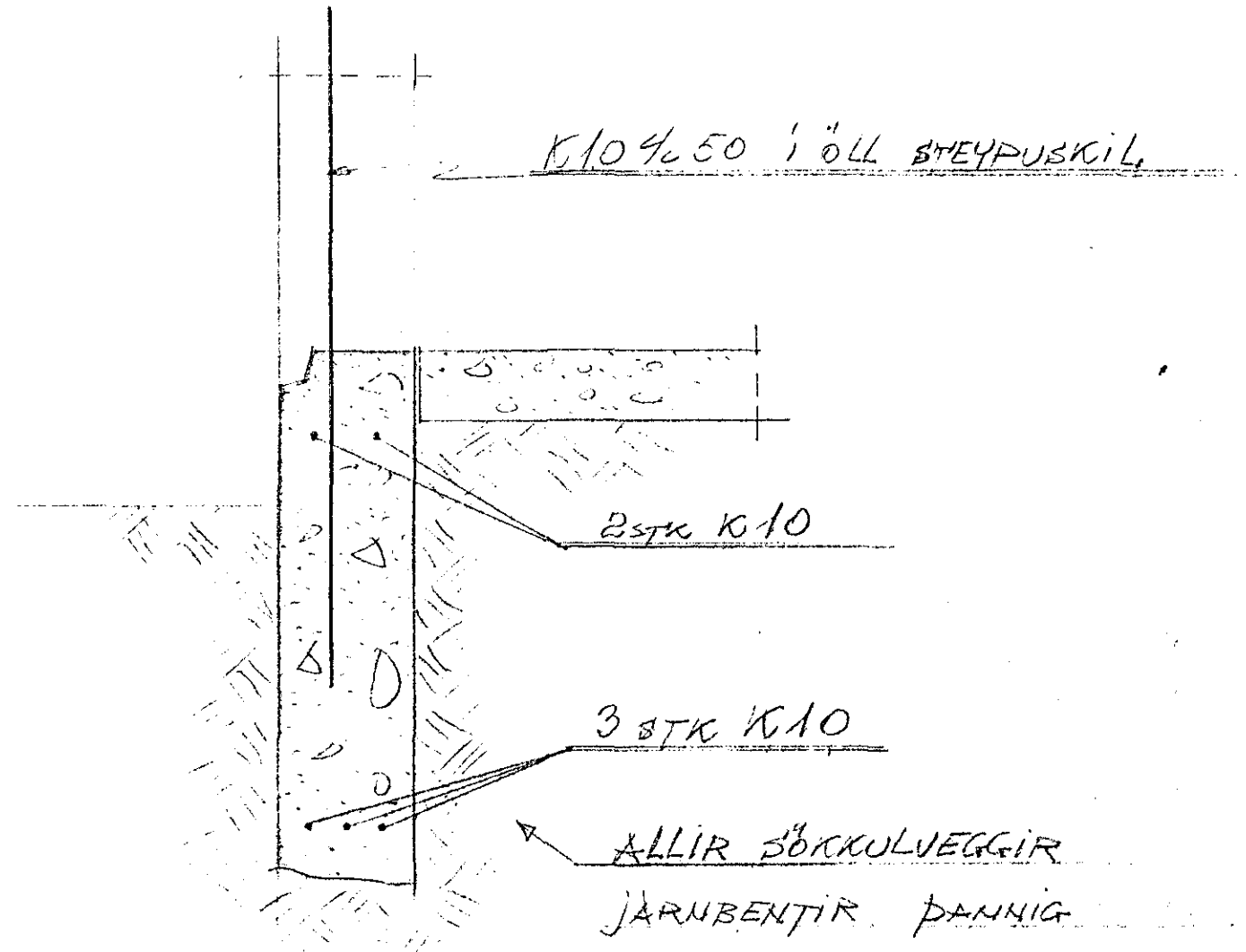
SNID I SÖKKULVEGG KVARDI 1:10
