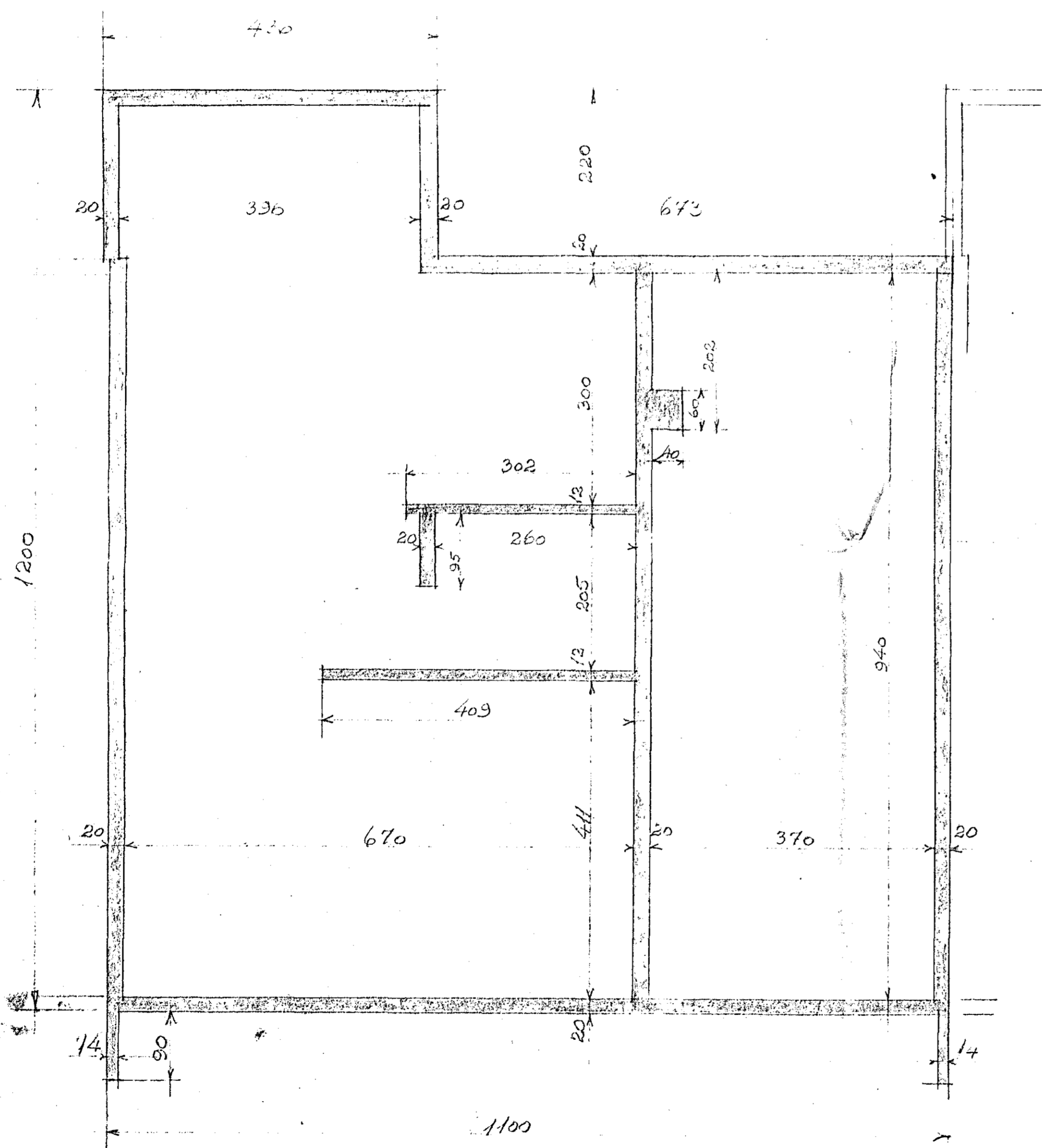
GRUNNMYND KVARDI 1:50
