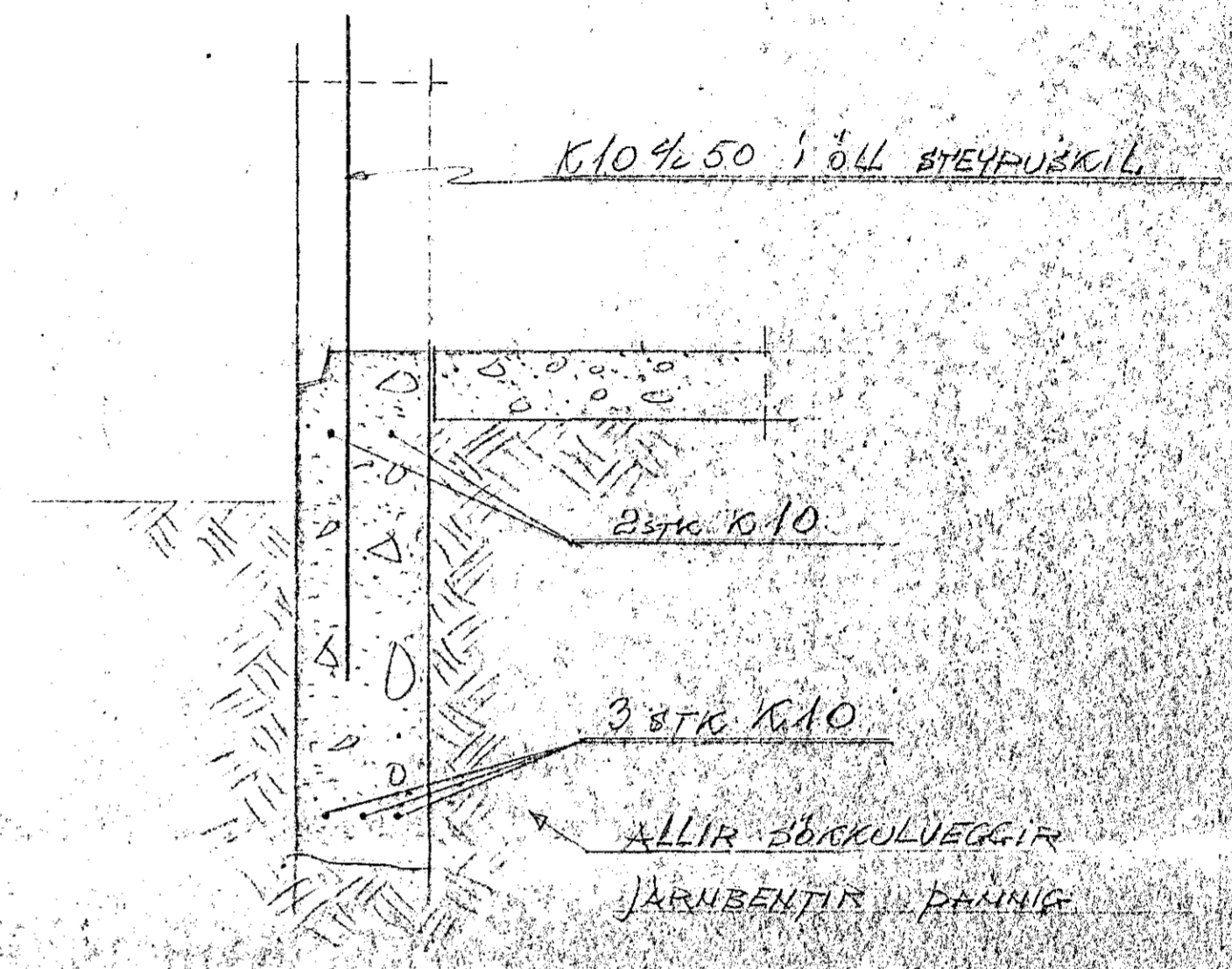
SNID I SÖKKULVEGG KVARDI 1:10
