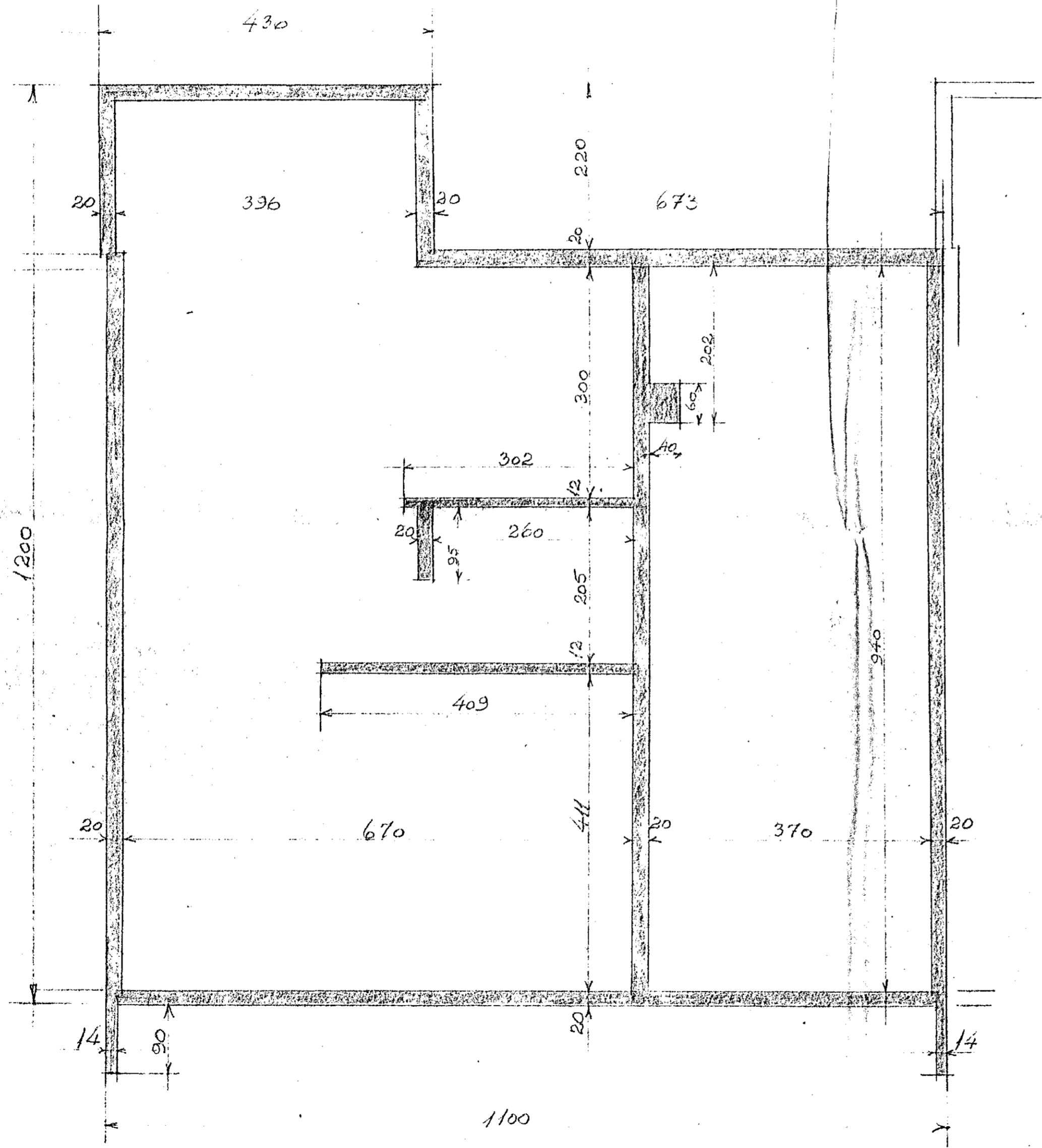
GRUNNMYND KVARDI 1:50
