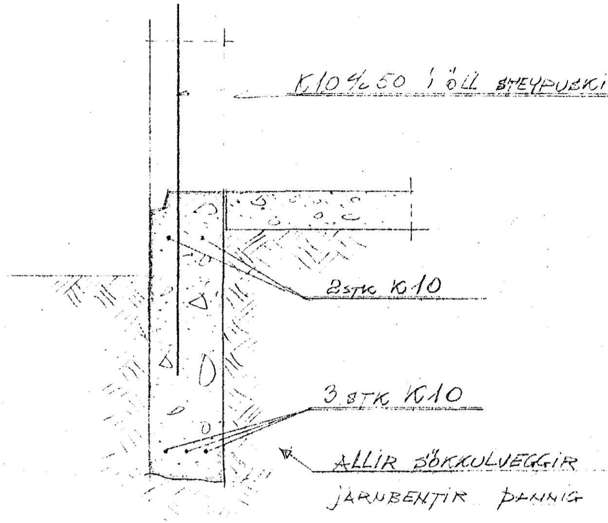
SNIÐ I SÖKKULVEGG KVARDI 1:10
