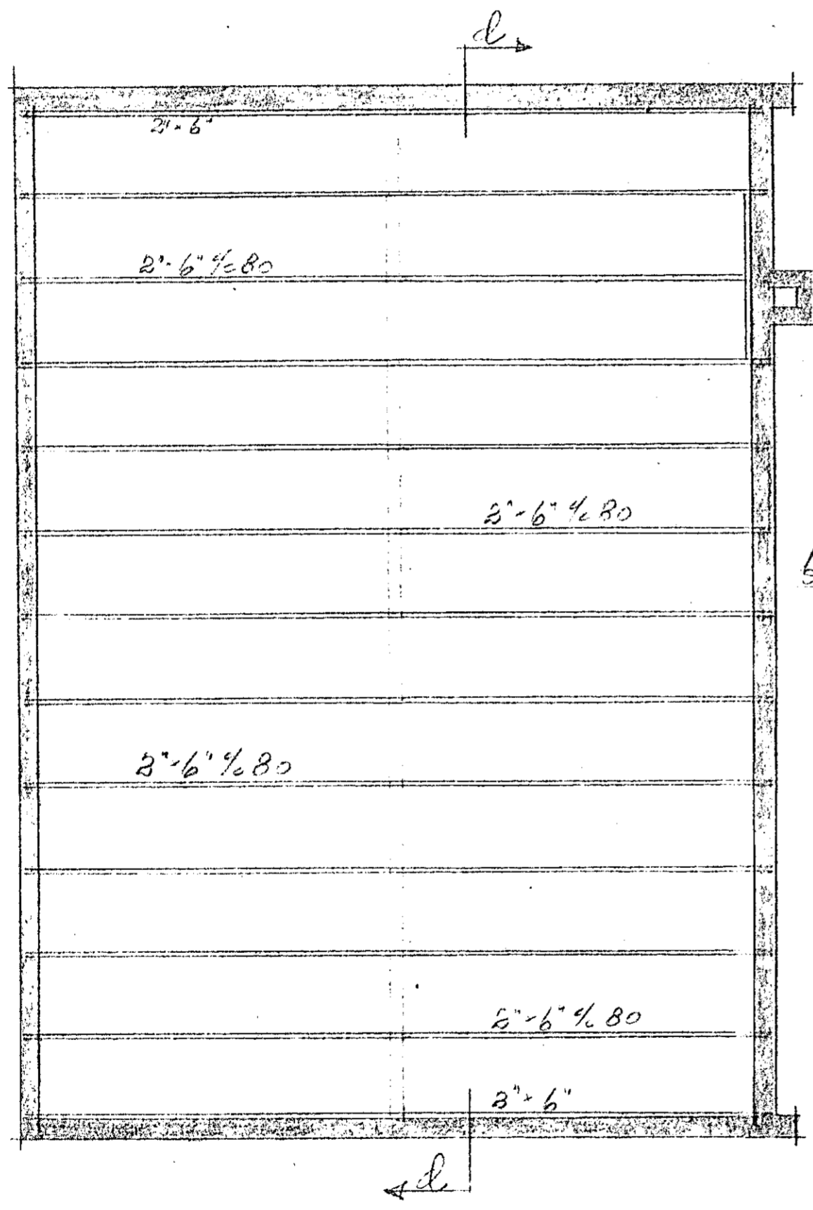
GRUNNMYND KVARDI 1:50
