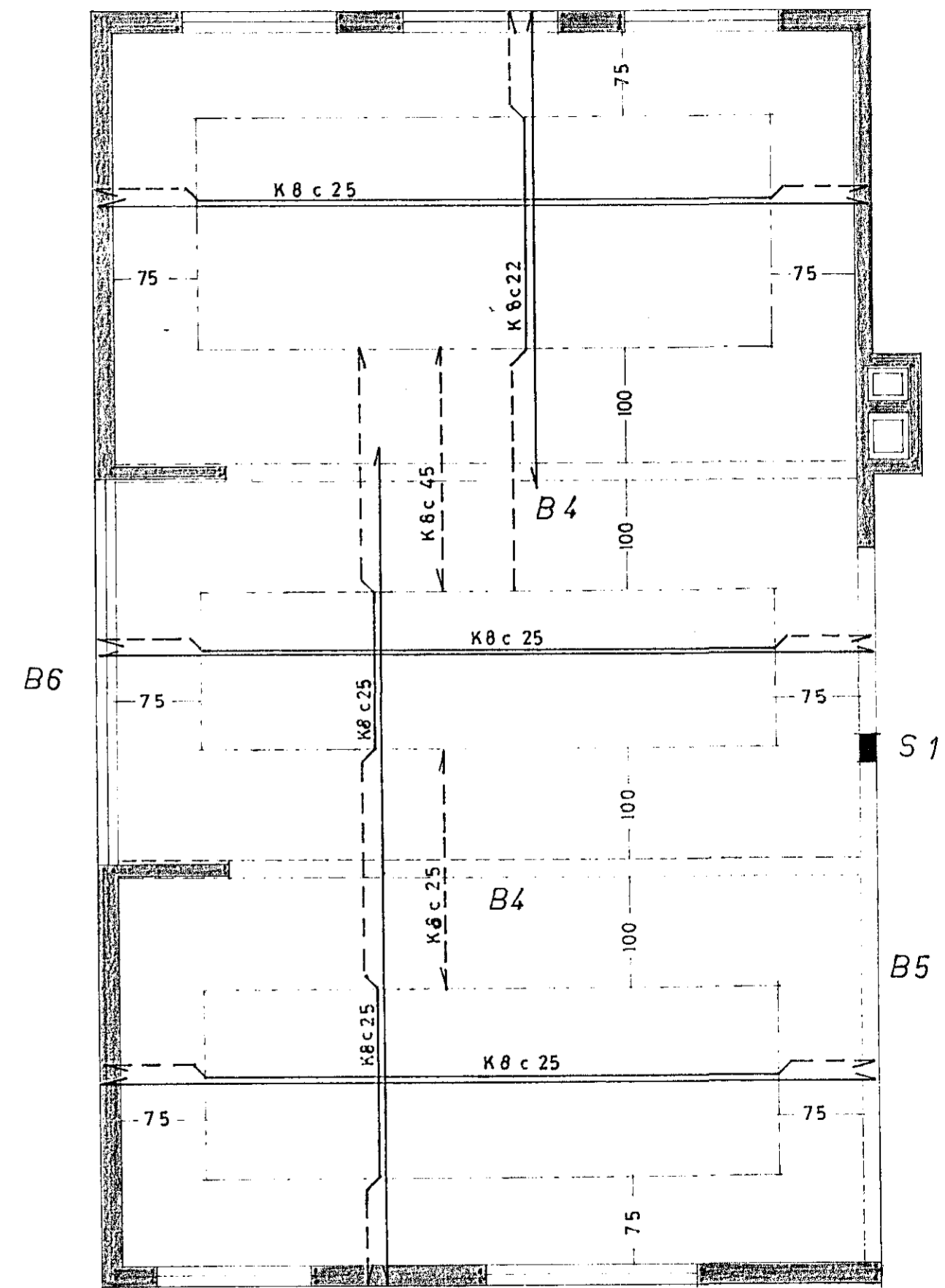
GRUNNMYND 2. HÆÐ
