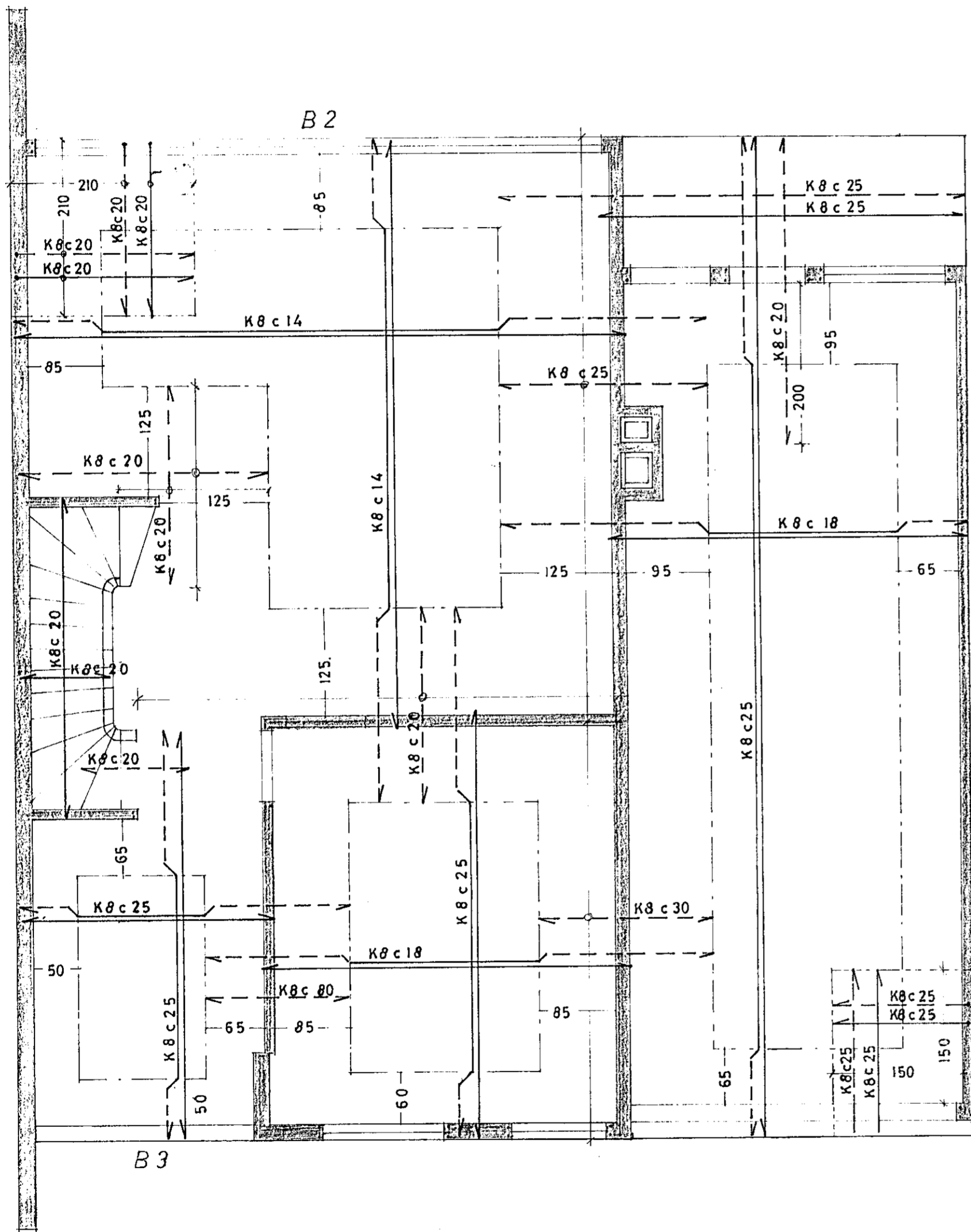
GRUNNMYND 1. HÆÐ
