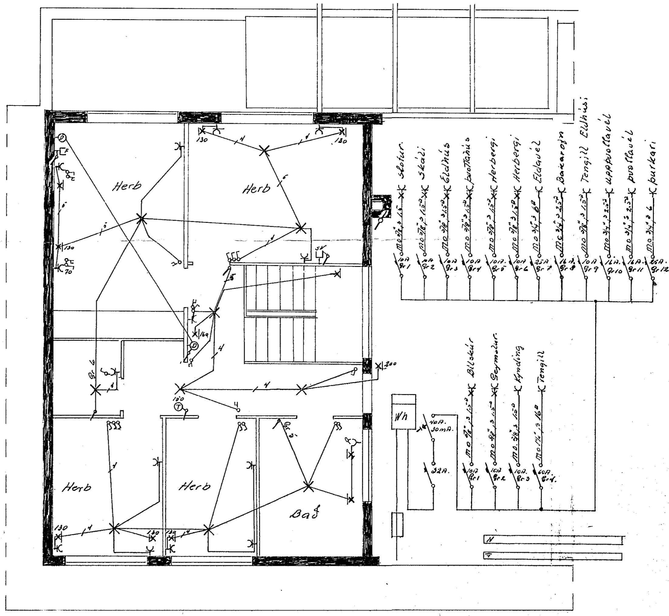
Miðvangur 125 Raflagnateikning bl. 1 af 1 Mál 1:50 Teiknað í sep. 1972 Jens Evertsson Sími 52829
