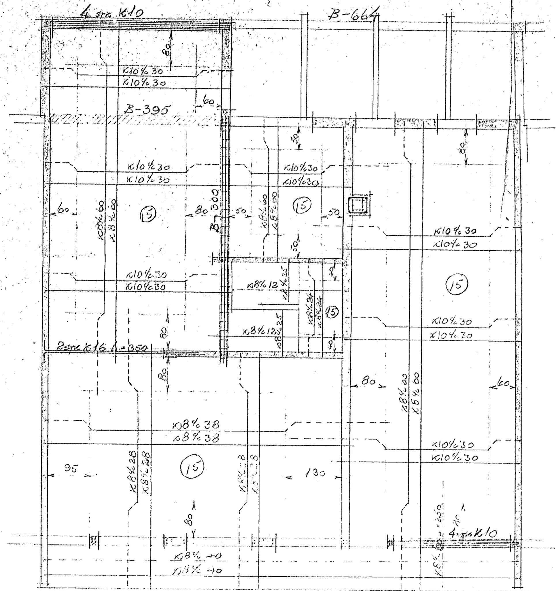
PLATA FÜR 1. HÆÐ
