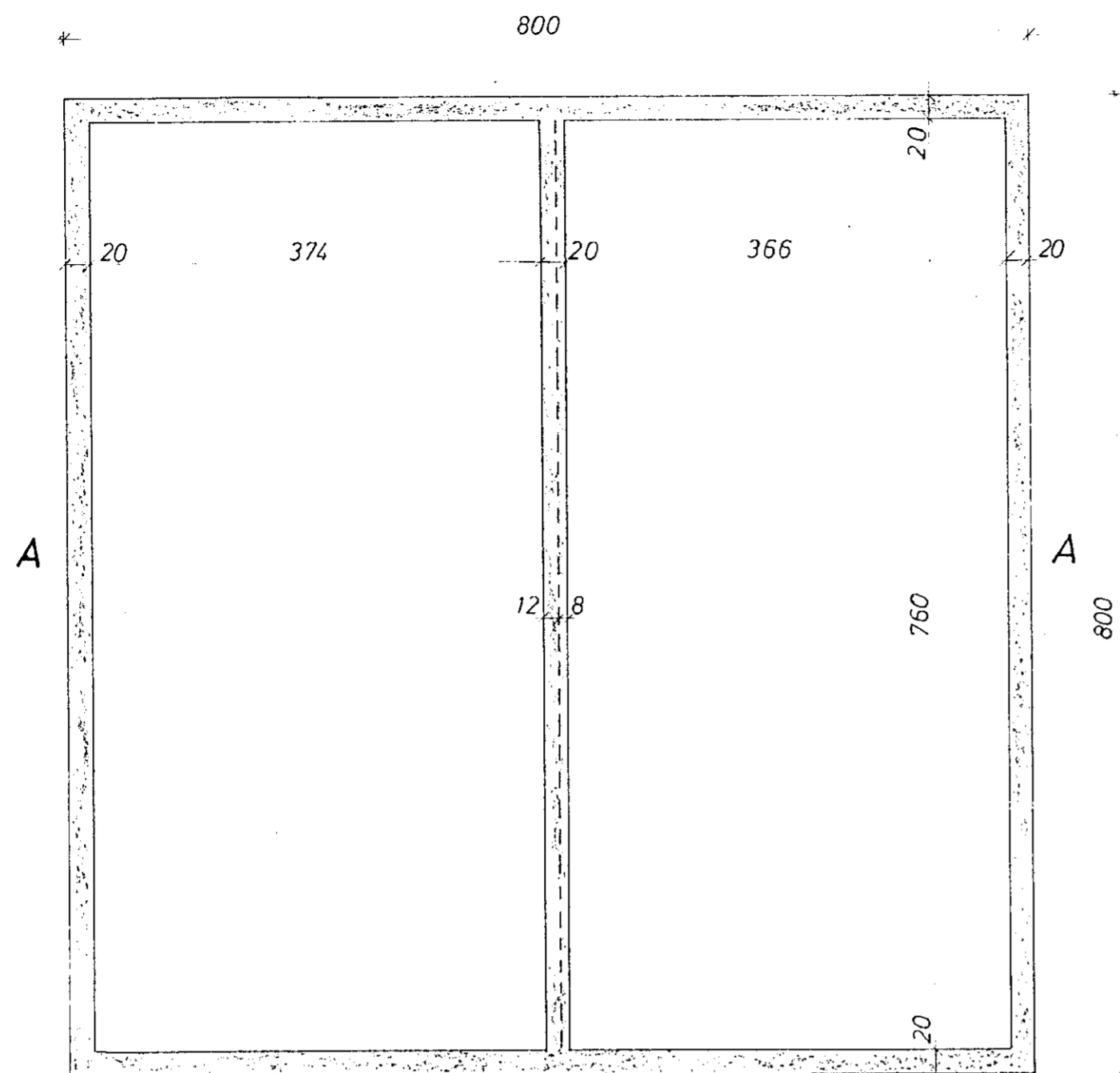
GRUNNMYND SÖKKLA 1:50
