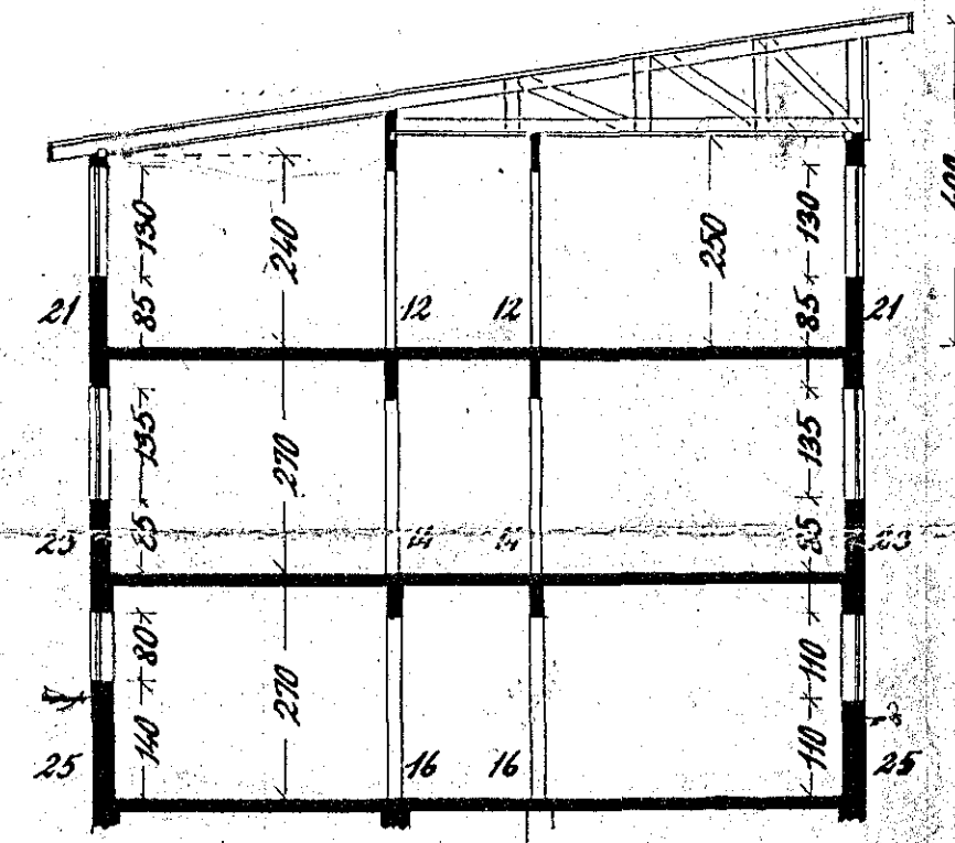
Þverskurður
