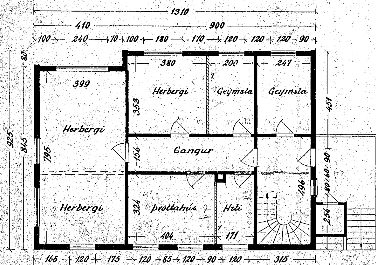
Kjallari
