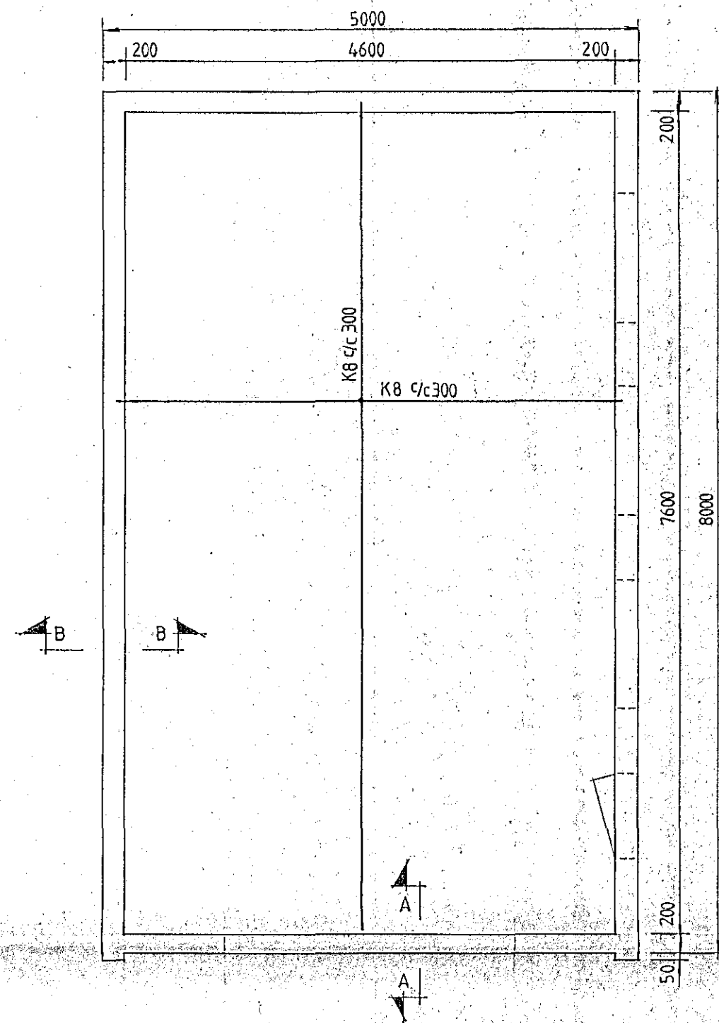
GRUNNMYND GÓLFLOTTU (1:50)
