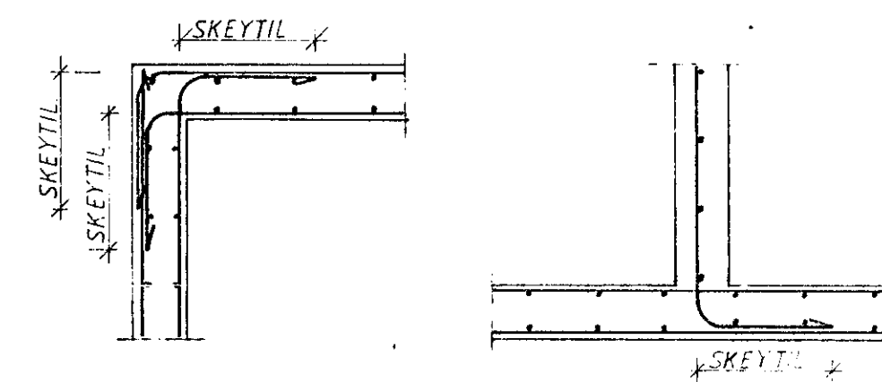
FRÄGANGUR JÄRNA NEMA ANNAD KOMI FRAM Á TEIKNINGUM.
