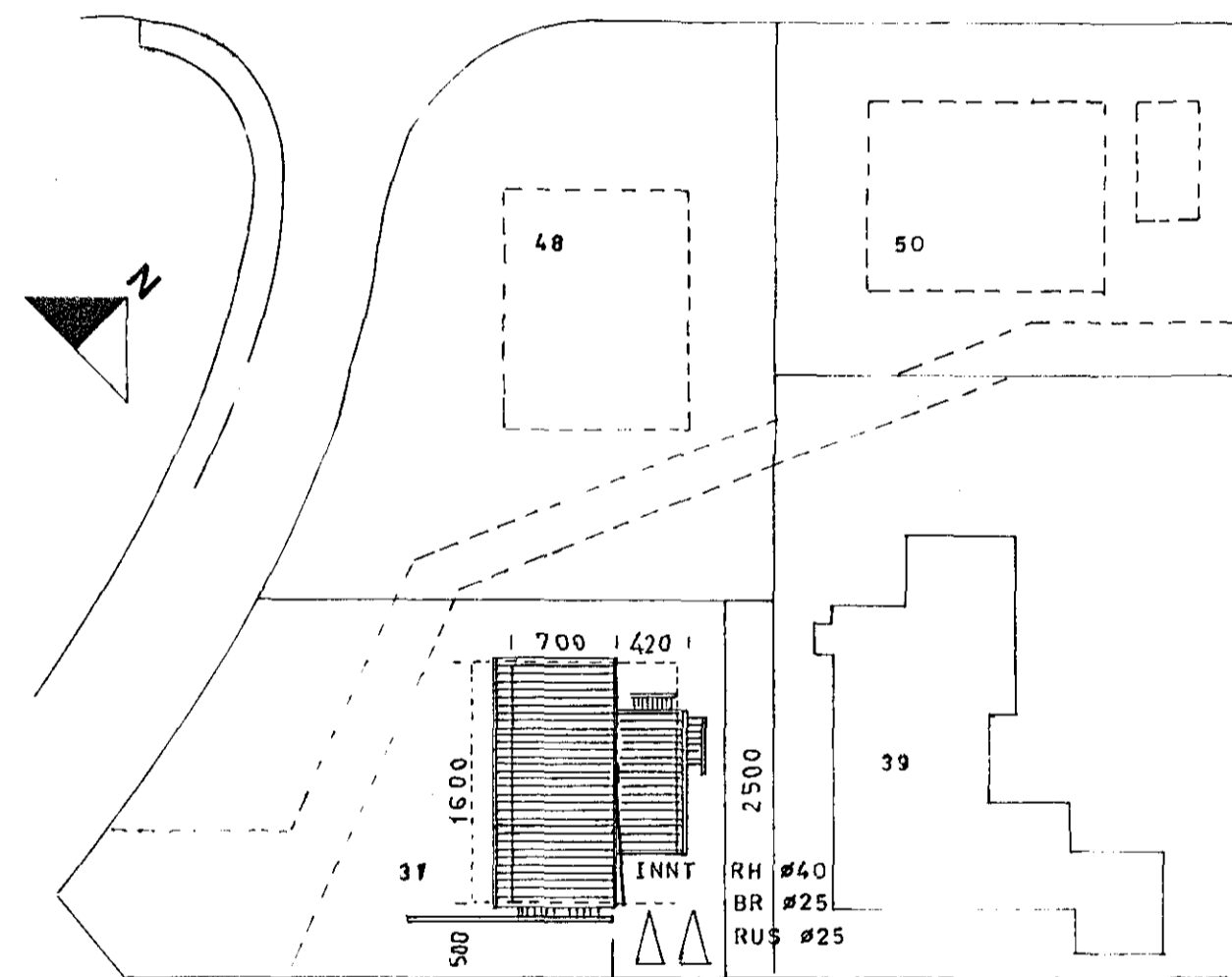
AFSTÖÐUMYND M 1:500
