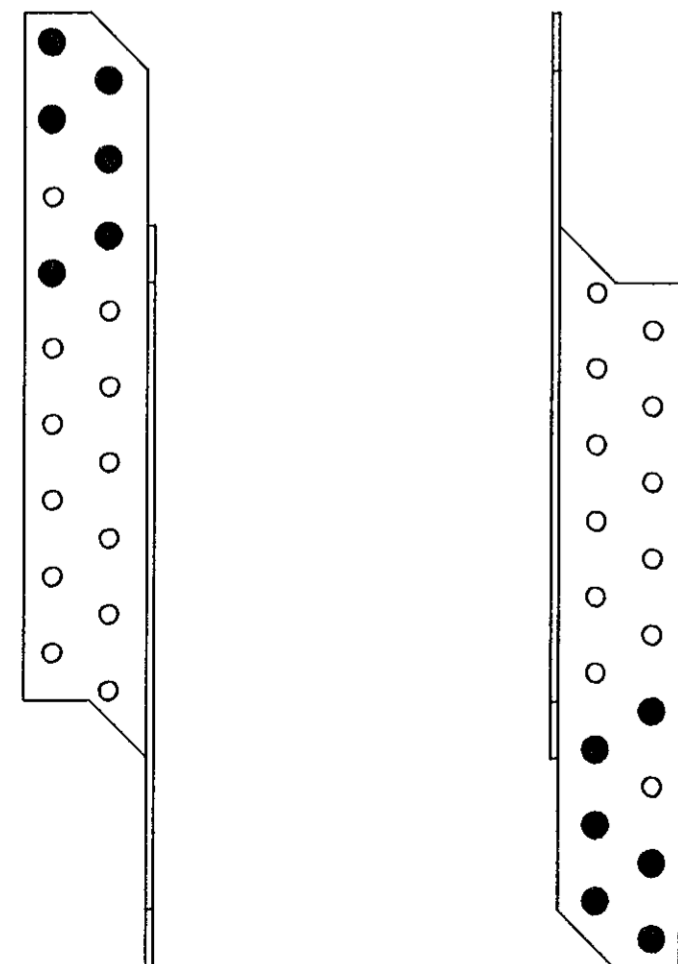
Hlið að sperru 6 stk BMF-kamsaumur 40/40
