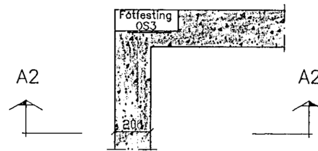
Sérmynd I S01 Mkv.1:20
