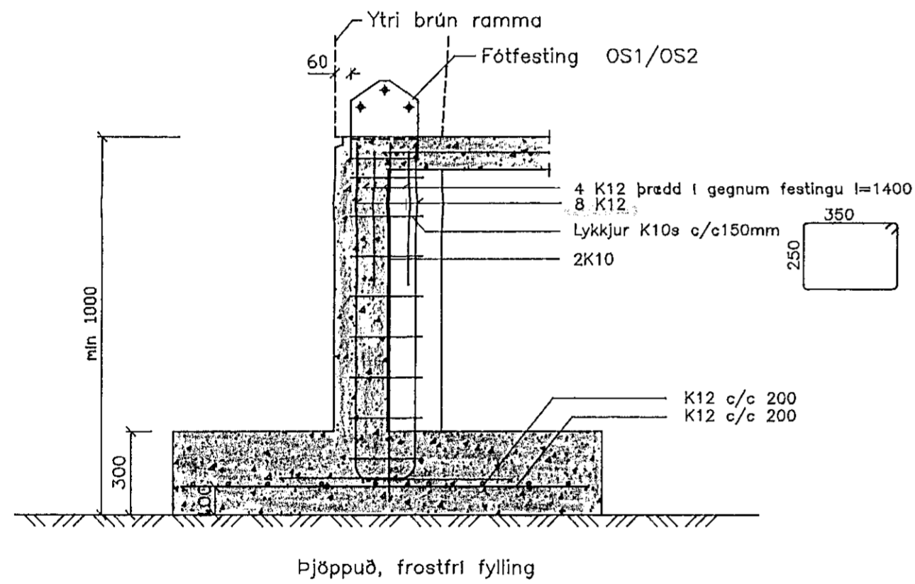
SNID A1-A1
