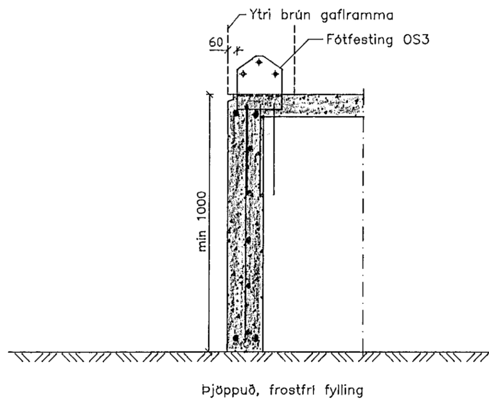
SNID A2-A2
