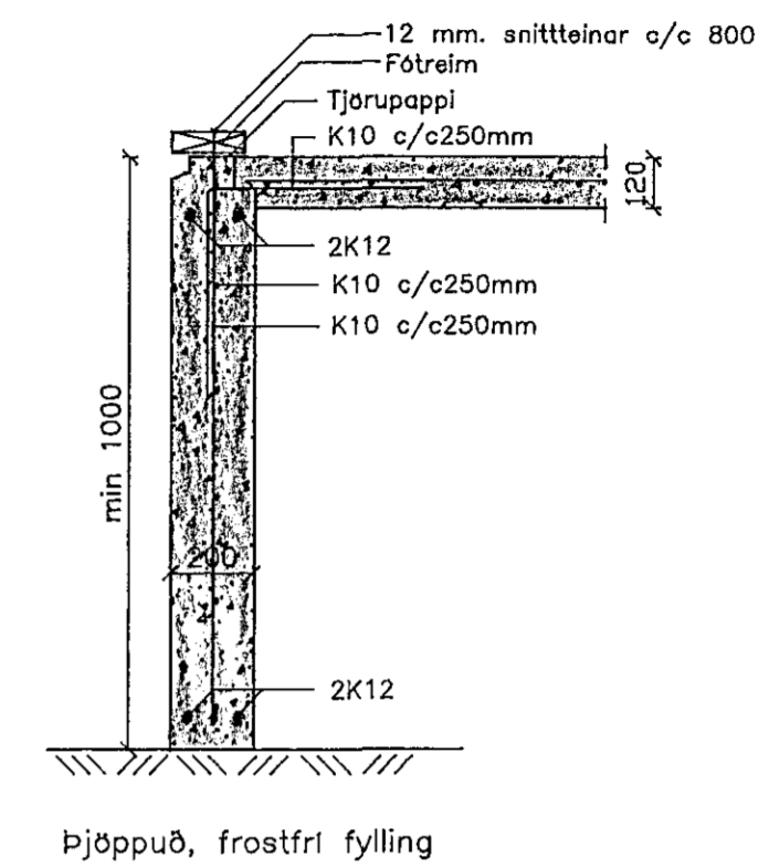
Snið I vegg IV S01 Mkv.1:20
