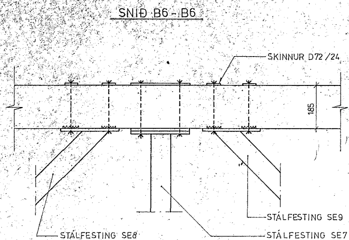
SNÍÐ B6 - B6
