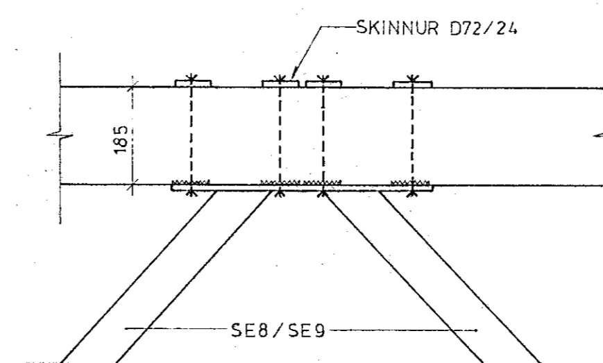
SNÍÐ A9 - A9
