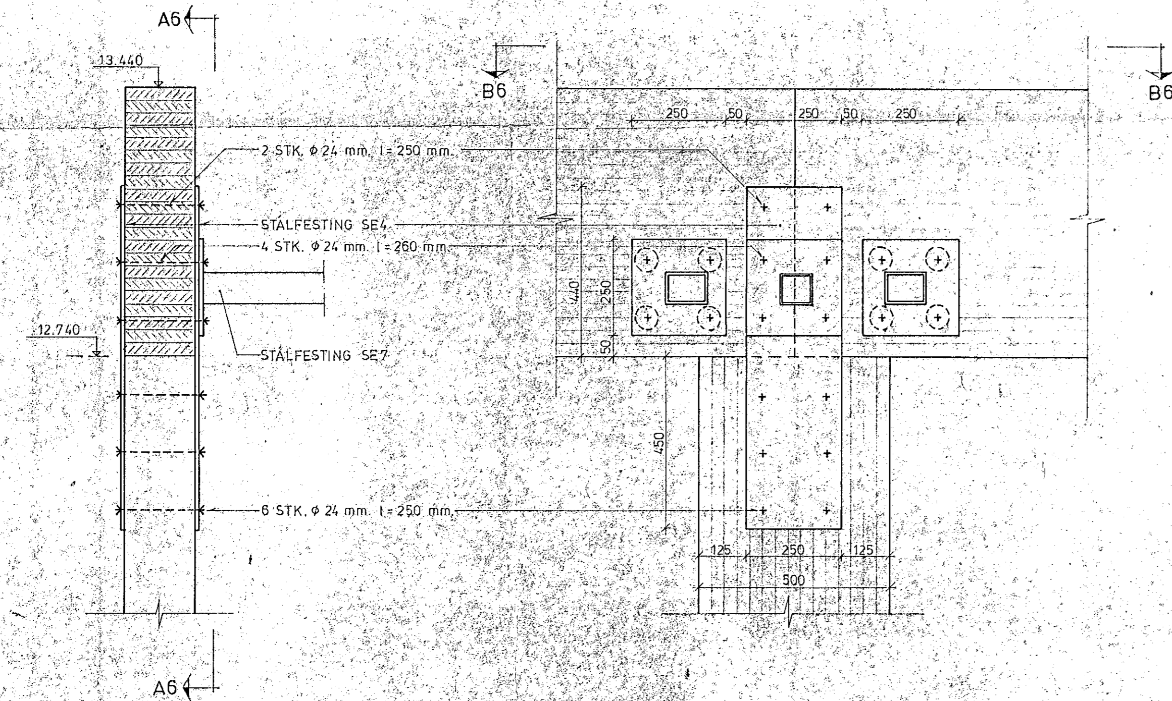
SNÍÐ B6 - B6
