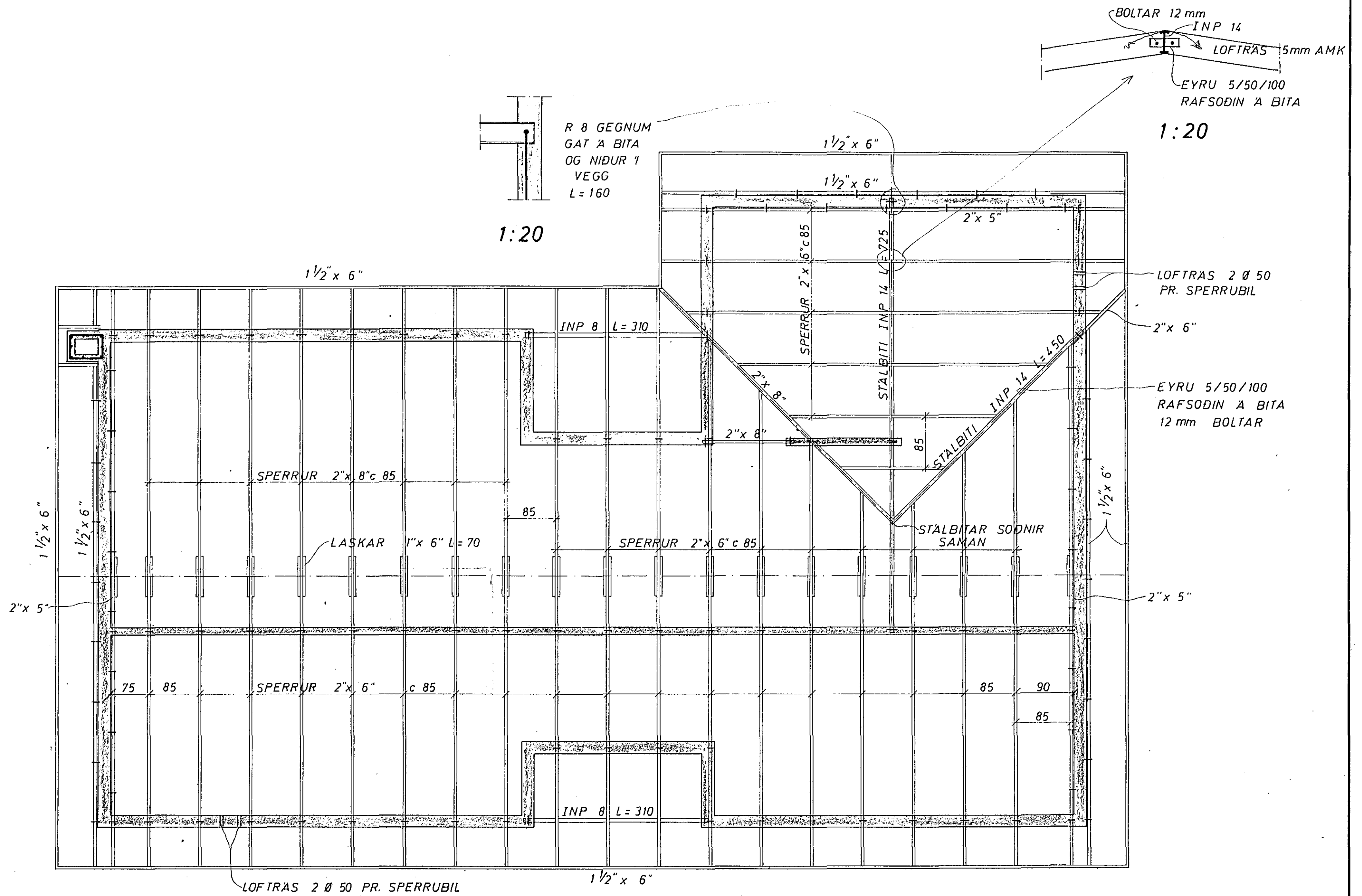
GRUNNMYND 1:50
